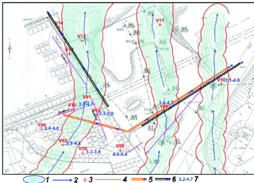
Рис. 7. Возможные варианты строительства дренажа для отвода грунтовых вод в районе строительной площадки: 1 – зоны увлажнения грунтов; 2 – направление миграции грунтовых вод; 3 – пункт ВЭРЗ; 4 – профили георадарного зондирования; 5 – вариант дренажной системы 1; 6 – вариант дренажной системы 2; 7 – глубины кровли и подошвы первого водоносного горизонта, м
