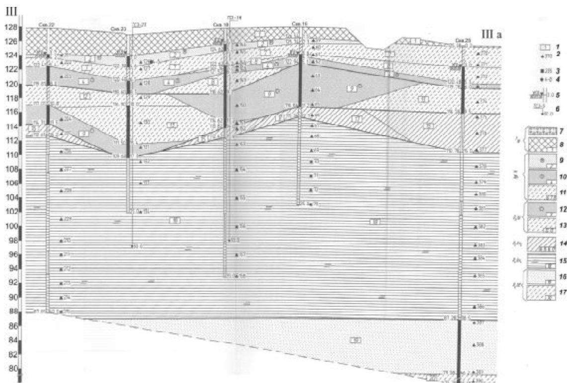
Рис. 2. Инженерно-геологический разрез по линии III–IIIa, построенный по результатам изысканий под строительство жилищного комплекса (ул. Краснопольская, 2-г, г. Киев): 1 – номер инженерно-геологического элемента; 2 – место отбора образца грунта нарушенного строения и его номер; 3 – место отбора образца почвы ненарушенного строения и его номер; 4 – место отбора пробы воды и ее номер; 5 – уровень грунтовых вод / дата измерения (глубина, м); 6 – точка статического зондирования, ее номер (глубина, м); 7 – почвенно-растительный слой с корнями растений (рекультивированный); 8 – насыпные пески пылеватые и мелкие, с прослойками супесей и суглинка, твердых, с включением строительного мусора 20–25 %, слежавшиеся; 9 – песок мелкий, желто-серый, от маловлажного до насыщенного водой, средней плотности; 10 – песок пылеватый, серый, желто-серый, насыщенный водой, средней плотности; 11 – супесь песчанистая, желто-серая, серая (6 – твердая, 7 – пластичная, 8 – текучая); 12 – песок пылеватый, темно-серый, зеленовато-серый, насыщенный водой, средней плотности; 13 – супесь песчанистая, темно-серая, зеленовато-серая (12 – пластичная, 13 – текучая); 14 – суглинок (“наглинок”) зеленовато-серый (14 – тяжелый пылеватый, твердый и полутвердый, 15 – тяжелый песчанистый, тугопластичный, 16 – легкий песчанистый, мягкопластичный, 17 – легкий песчанистый, текучепластичный и текучий); 15 – глина легкая пылеватая (“киевский мергель”) зеленовато-серая, полутвердая и тугопластичная, очень редко твердая, с тонкими, 1–3 см, прослойками песка пылеватого 15–20 %; 16 – песок от мелко- до среднезернистого, зеленовато-серый, глауконитовый, плотный, насыщенный водой, слабосцементированный; 17 – супесь песчанистая, зеленовато-серая, глауконитовая, текучая, слабосцементированная
