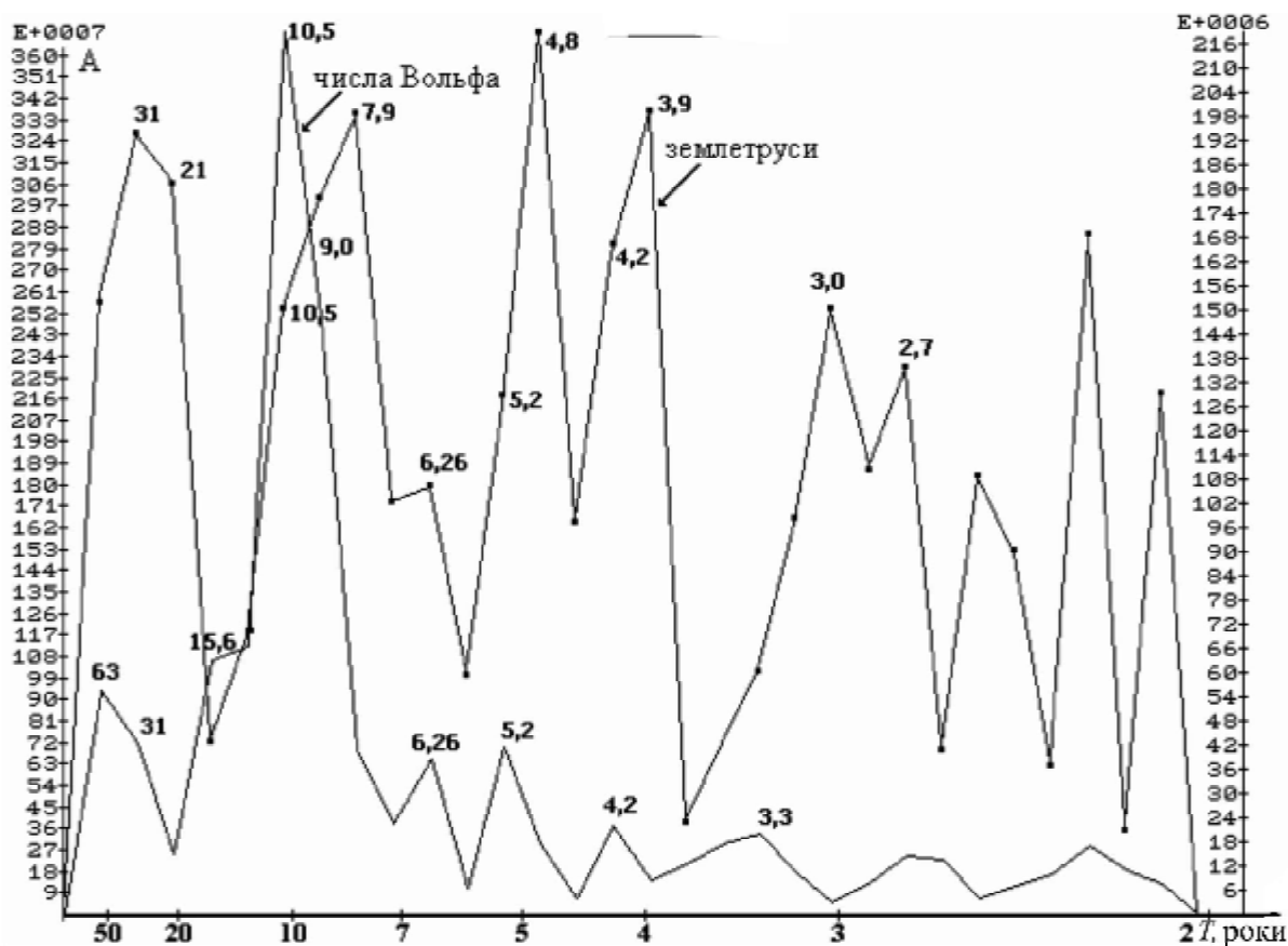
Рис. 3. Спектри (періодограми) варіацій сонячної активності (чисел Вольфа) і сейсмічної активності (кількість землетрусів) за 1961–2004 рр. у Карпатському регіоні України (шкала X – спектральний період варіацій, у роках; шкали Y – в умовних одиницях)
