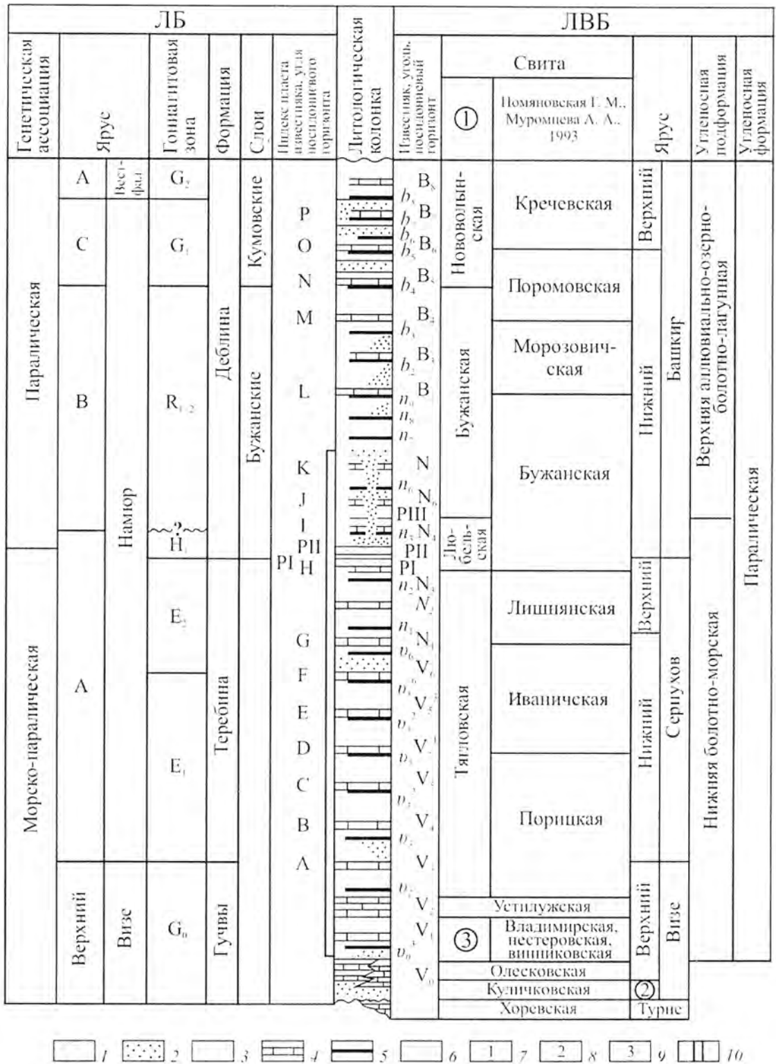
Рис. 2. Положение глубоких горизонтов и угольных пластов в стратиграфическом разрезе карбона польско-украинской части Львовско-Люблинского бассейна
