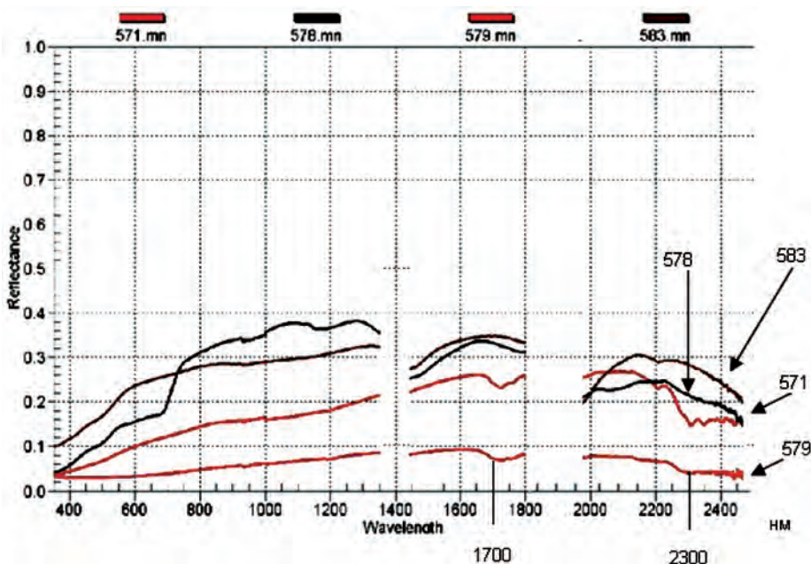
Рис. 3. Зіставлення спектрів відбиття нафтонасичених ґрунтів (точки 571, 579), сухого ґрунту (точка 578) та зволоженого суглинку (точка 583) над нафтовим родовищем
