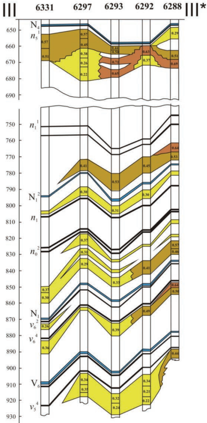
Рис. 4. Літолого-стратиграфічний розріз з викидонебезпечною ситуацією по профілю III–III* (за матеріалами [Забигайло и др., 1990])
