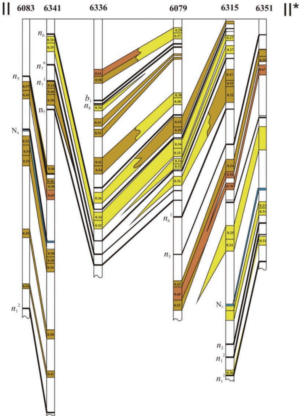
Рис. 3. Літолого-стратиграфічний розріз з викидонебезпечною ситуацією по профілю II-II* (за матеріалами [Забигайло и др., 1990]) Умов. позначення див. на рис. 2
