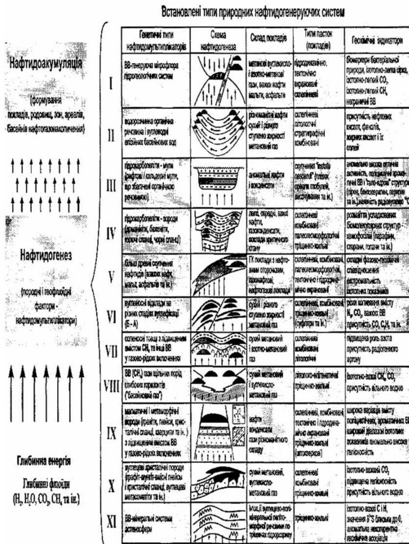
Рис. 2. Принципова схема нафтидогенезу і типи природних нафтидогенеруючих систем Fig. 2. Principal scheme of naftidogenesis and types of natural naftidogenerating systems
