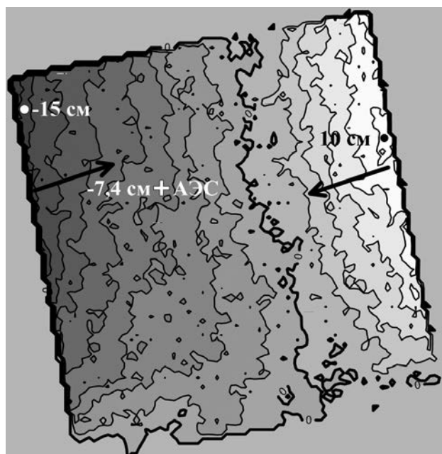
Рис. 5. Горизонтальные смещения земной поверхности по результатам радарной съемки ИСЗ ERS2(18.08.1997 – 05.04.1999). Изолинии нанесены через 2 см
