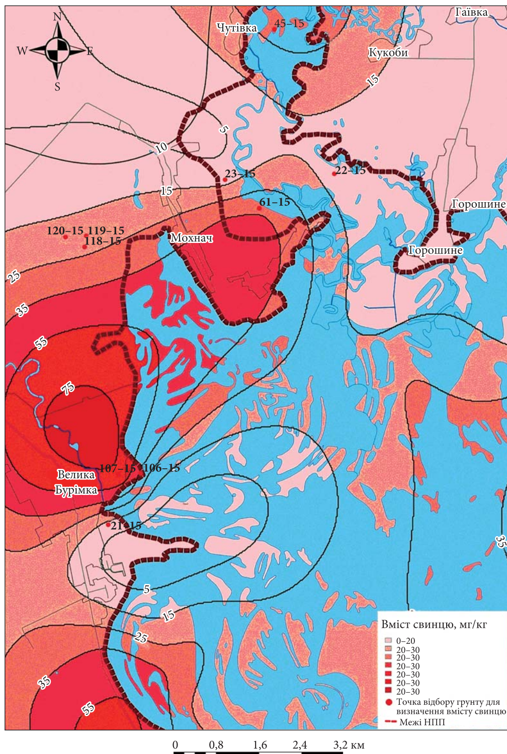
Розподіл свинцю у сучасному ґрунтовому покриві території НПП “Нижньосулський” Lead distribution in the modern soil cover of the territory of National Nature Park “Nyzhnyosulskyi”
