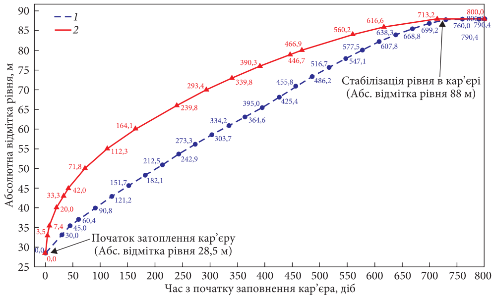
Рис. 4. Динаміка підйому рівнів води в кар'єрі Стильський під час його «мокрій» консервації за даними моделювання: 1 — графік підйому рівнів води в кар'єрі Стильський за схемою «великого колодязя» без перерахунку для реальної геометрії кар'єру; 2 — графік підйому рівнів води в кар'єрі Стильський з урахуванням реальної геометрії кар'єру (приведені значення)
