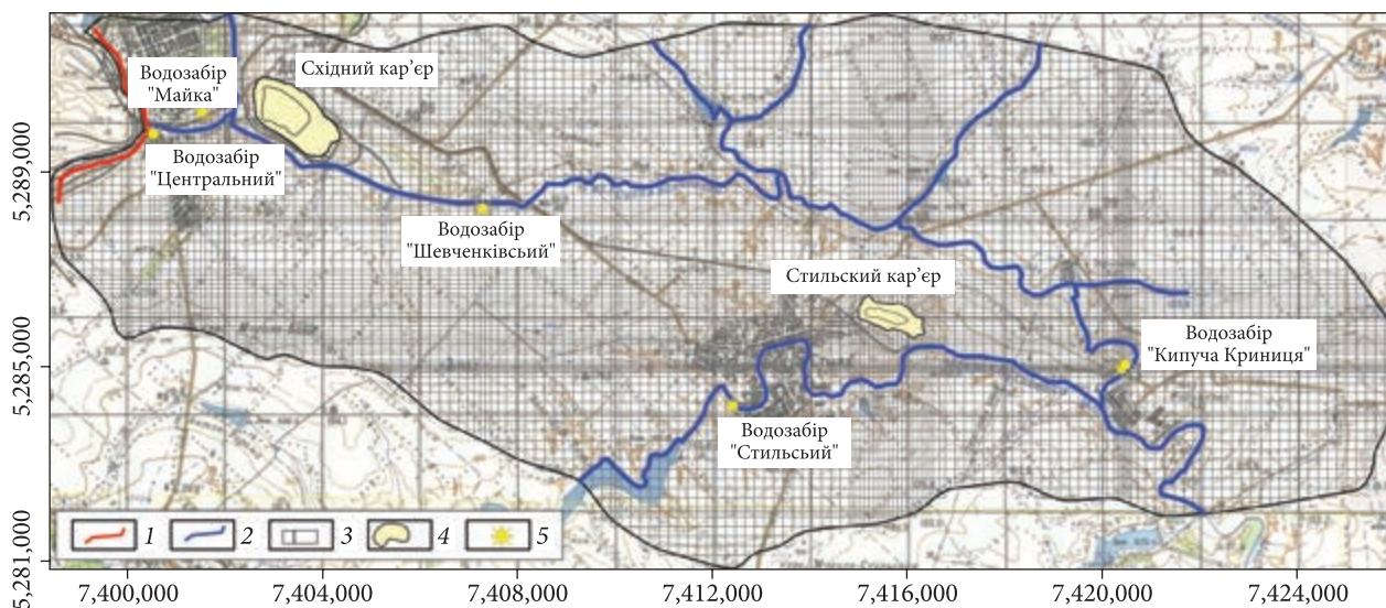
Рис. 1. Карта граничних умов і просторової дискретизації моделі: 1 — гранична умова (ГУ) I роду (фіксований рівень, що змінюється в часі); 2 — гранична умова «річка» (ГУ III роду); 3 — модельні блоки просторової дискретизації області фільтрації; 4 — територія кар'єрів — фіксований рівень, що змінюється в часі, ГУ I роду H = f(t) ; 5 — водозабори — гранична умова II роду (фіксований дебіт, що змінюється в часі)
