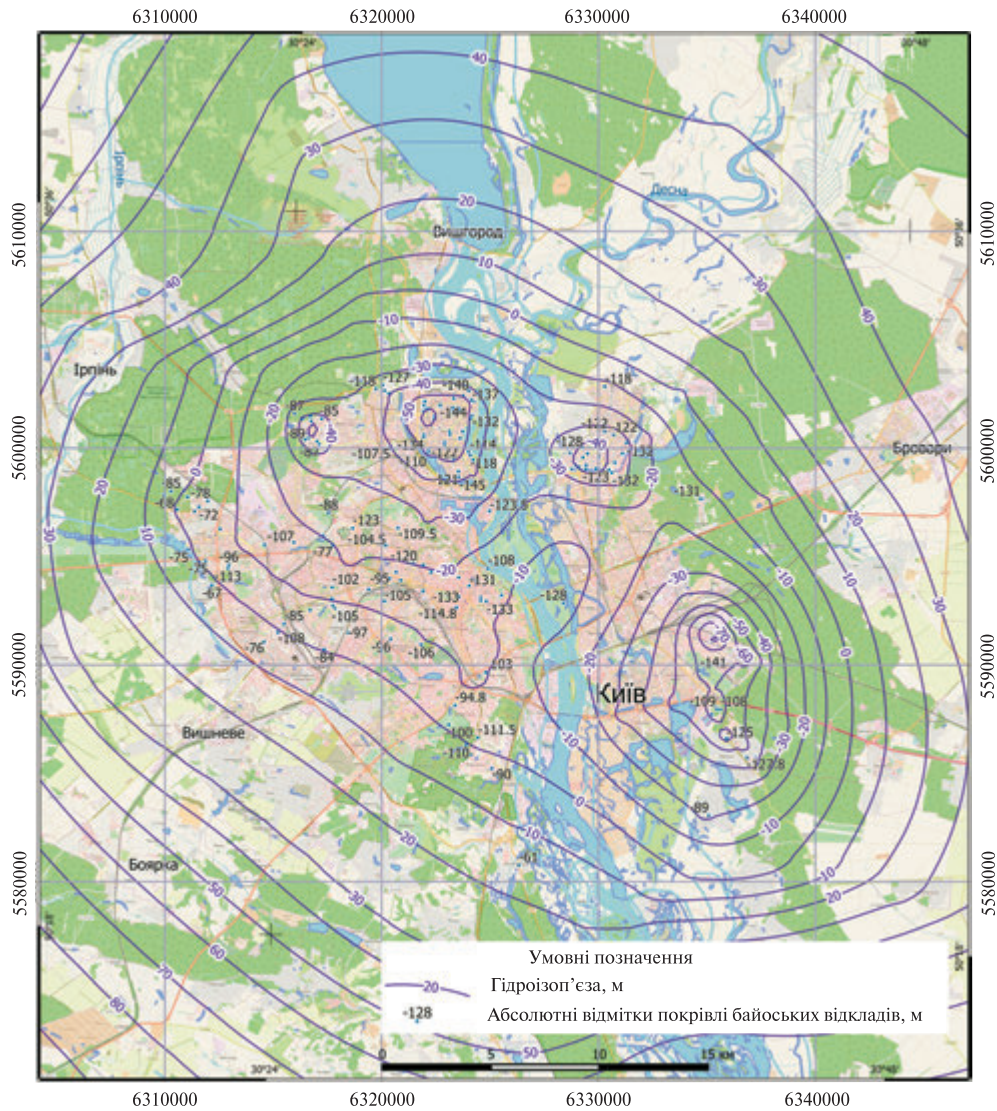
Рис. 9. Карта гідроізоп'єз байоського водоносного горизонту за результатами розв'язання другого варіанту прогнозу станом на 2043 р. Fig. 9. Map of the hydroisopiestic lines for the Bajocian aquifer based on the results of the 2nd scenario of the model forecast as of 2043
