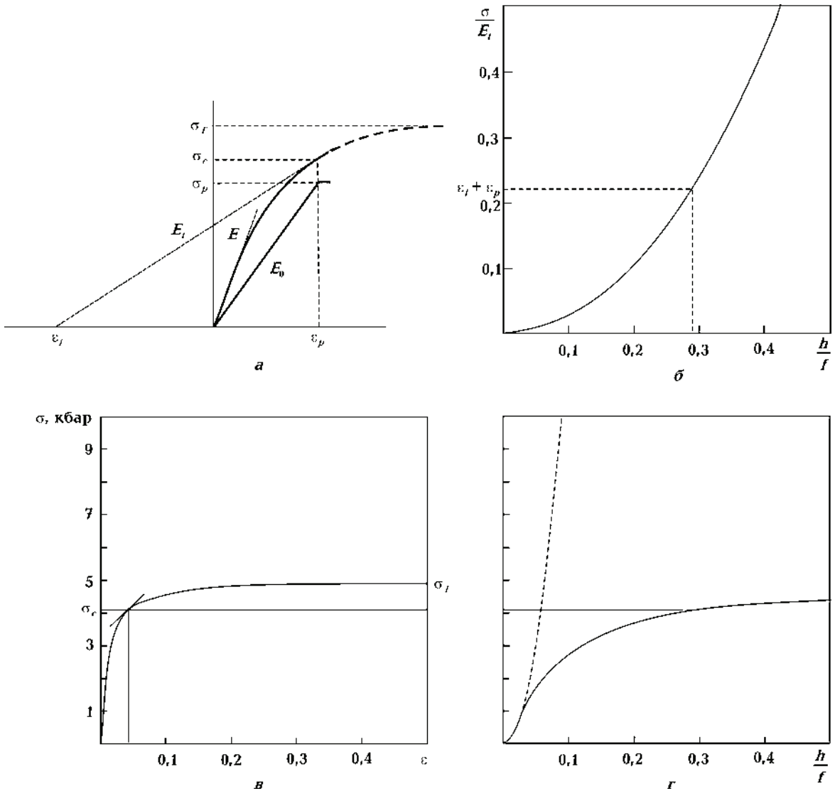
Рис.3. К определению изгиба за пределом упругости: a — схема расчета касательного модуля, поясняющая также суть прочностного критерия: одновременность достижения критического изгибного напряжения \sigma_c в слое и предела прочности вмещающей среды \sigma_p ; \sigma_T — предел текучести слоя; б — диаграмма изгиба за пределом упругости; в — эмпирическая кривая деформирования (уравнение (4)). Отмечено состояние потери изгибной устойчивости, контролируемое касательным модулем деформации [Вольмир, 1967; Пановко, Губанова, 1987]; г — связь критического напряжения с относительной мощностью при одиночном изгибе, полученная на основе (7). Штриховая линия — кривая Эйлера.
