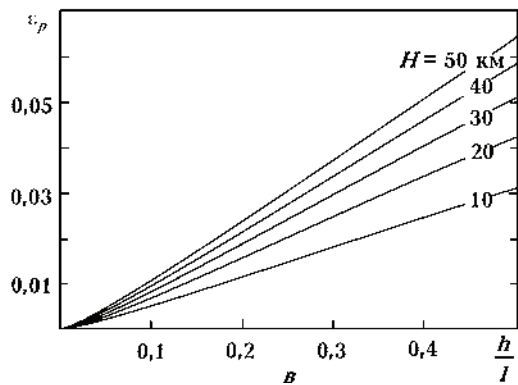
Рис. 4. Связь изгибной складчатости с глубиной и величиной доскладчатой деформации: а — относительной мощностью одиночного изгиба в функции глубины; б — модели изгиба слоя постоянной мощности на разных глубинах (на основе рис. 5, а); в — кривые связи относительной мощности с величиной деформации на начало изгиба.
