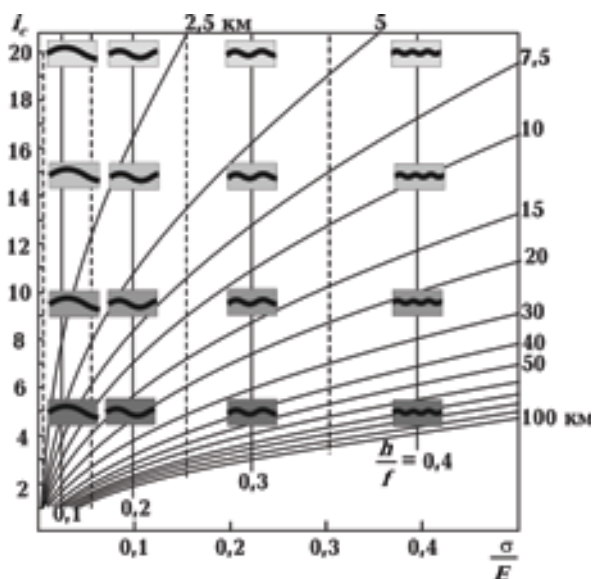
Рис. 6. Прогноз развития изгибной складчатости одиночного слоя в зависимости от глубины и контраста свойств слоя и среды в прочностном приближении. Показаны изолинии относительной мощности и глубины (км), а также модели складчатости изгиба одиночного слоя в среде с различным индексом компетентности (фон).
