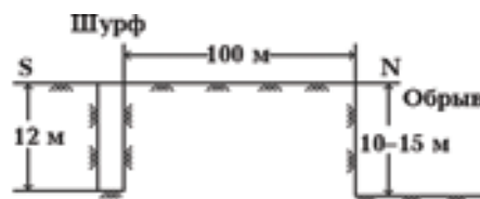
Рис. 1. Схема рельефа вблизи геофизического шурфа на станции "Березовая Рудка". 31.10.1972 г.
