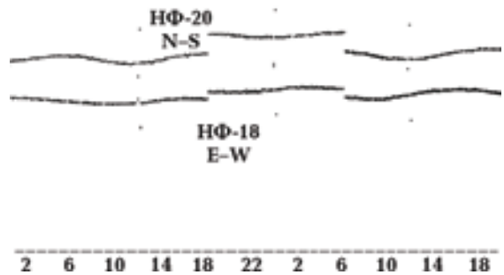
Рис. 2. Фрагмент записи наклонов земной поверхности в момент приложения и снятия нагрузки вблизи шурфа. Станция "Березовая Рудка". 31.10.1972 г.
