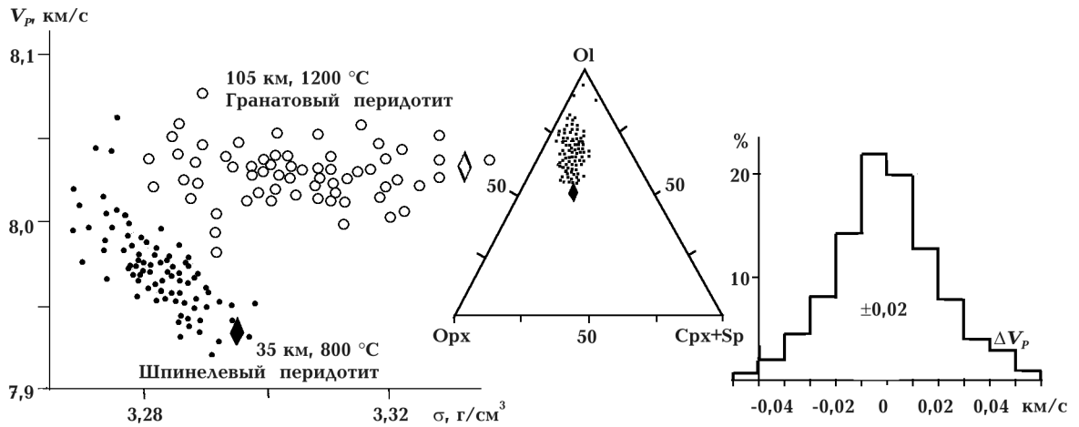
Рис. 3. Значения скорости распространения продольных волн и плотности мантийных пород разного состава [Sobolev et al., 1996] и гистограмма изменчивости скорости. Ромбы — данные для примитивной мантии.
