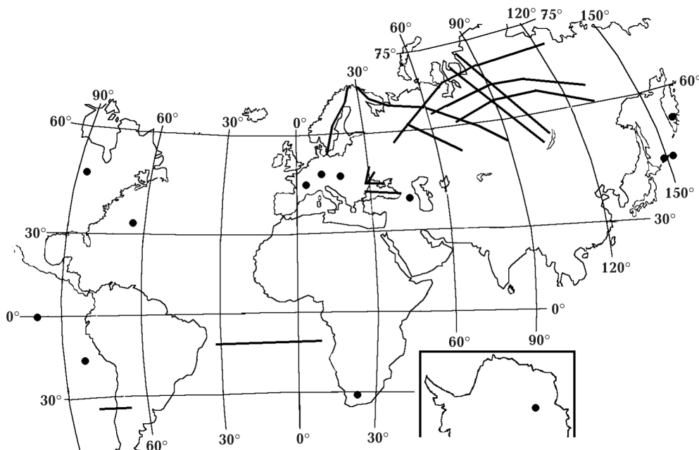
Рис. 7. Размещение использованных экспериментальных скоростных разрезов. Линии — региональные геотравессы, точки — места локальных моделей. На врезке — Антарктида.
