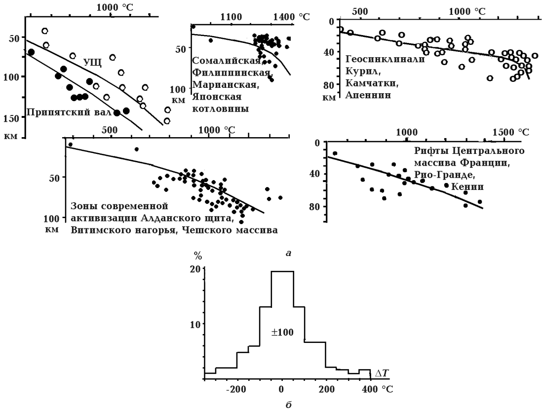
Рис. 5. Тепловые модели и данные геотермометров (а)[Ащепков и др., 2001; Глебовицкий и др., 2001; 2003; Доусон и др., 1997; Медарис и др., 2000; Тектоносфера ..., 1992; Уханов и др., 1988; Фролова и др., 1989; Цымбал, 2003; Цымбал и др., 1996; Bryant et al., 2006; Coltorti et al., 1999; Jones et al., 2000; Sobolev et al., 1996 и др.] (линии — расчетные температуры, точки — экспериментальные); гистограмма различий расчетных и экспериментальных данных (б).
