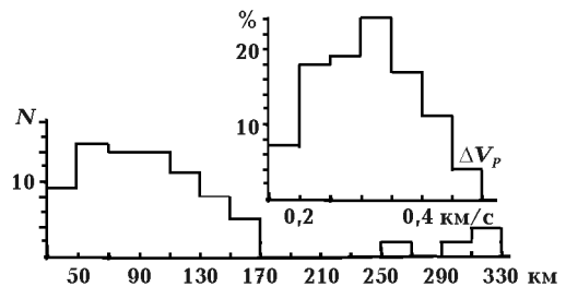
Рис. 11. Распределение по глубине количества аномальных отклонений экспериментальных величин V_p от расчетных ( N — точки на рис. 8, 9) и гистограмма распределения их интенсивности.
