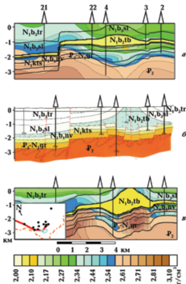
Рис.9. Разрез пространственной геоплотностной модели Солотвинского газового месторождения по линии скважин 21, 22, 4, 3, 2: а — при использовании неправильной формы соляного тела; б — геологическая модель по [Лозиняк, Малевич, 2005]; в — полученный после уточнения формы соляного тела.
