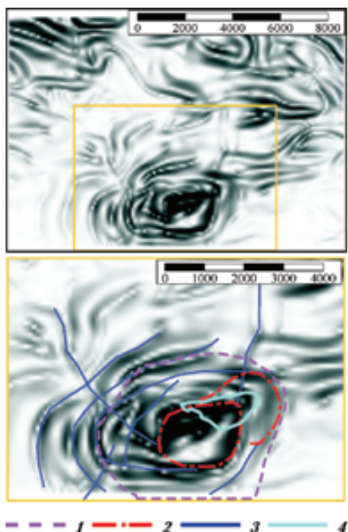
Рис. 10. Выделение приштоковых тектонических нарушений на основе анализа остаточной компоненты гравитационного поля: 1 — внешний контур соляного тела; 2 — внутренние контуры опущенного и приподнятого блоков в подошве соляного тела; 3 — тектонические нарушения; 4 — контур выхода соляного тела на дневную поверхность (Петрашкевич Н.И., Лозиняк П.Ю.).
