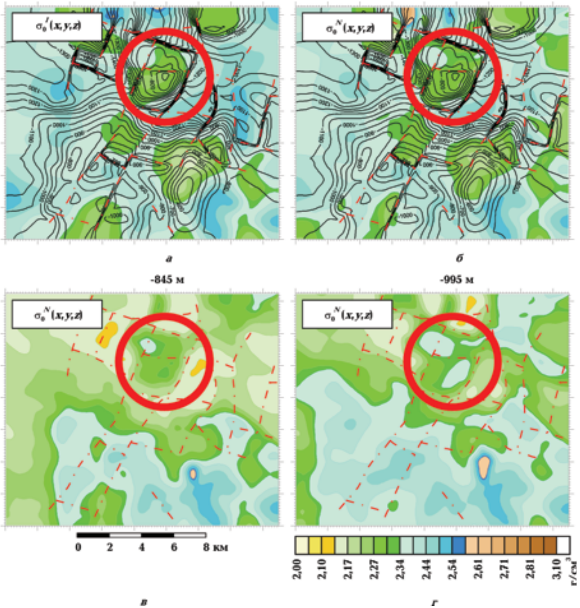
Рис. 7. Сопоставление распределения плотности в куполе структуры доробратовской свиты сармата N_{1s,dr} : а, б — внутрипластовые срезы моделей на основе пространственно информативных данных и пространственно низкоинформативных данных соответственно; в, г — горизонтальные срезы модели на основе пространственно низкоинформативных данных на уровнях -845 и -995 м.
