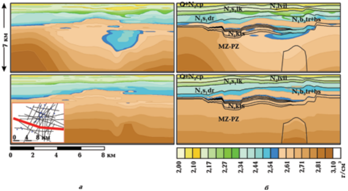
Рис.5. Разрез по линии синтетического профиля. Априорная геоплотностная модель (внизу) и результат решения обратной линейной задачи гравirazведки (вверху) для модели на основе пространственно низкоинформативных (2D+1D) (а) и пространственно информативных (3D+2D+1D) (б) данных.
