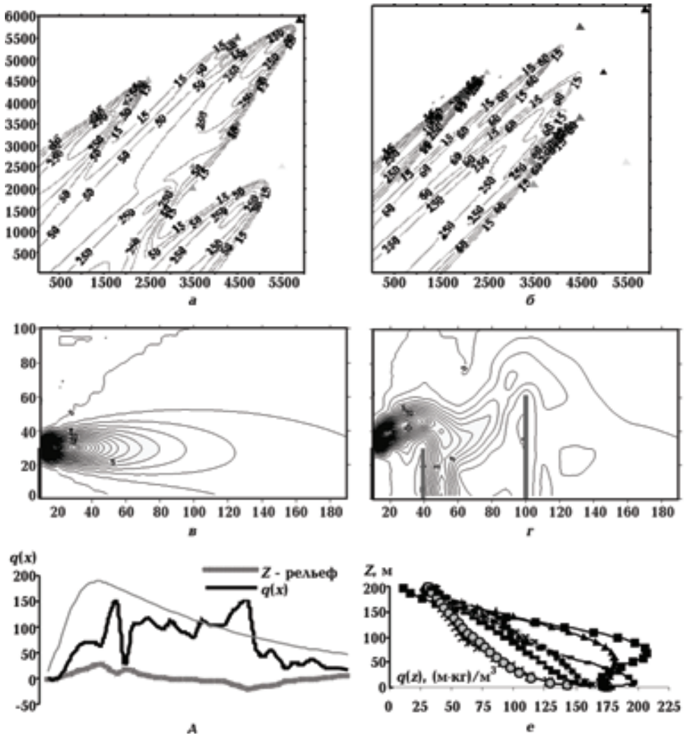
Рис. 1. Распределение q(x, y, z) , рассчитанное с помощью модели МЛАД: a, б — суммарное поле q(x, y) SO_2 от 9 источников; в, г — распределение q(x, z) над ровной и городской поверхностью; д — распределение q(x) над сложным рельефом; е — профили q(z) , k_z = \phi(z) на расстоянии x \approx x_{max} (все концентрации в мкг/м^3 ).
