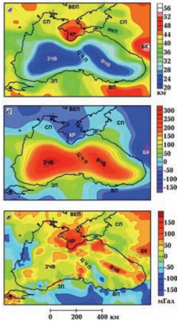
Рис. 6. Поверхность Мохо (а), ее гравитационный эффект (б) и разностное гравитационное поле II Черноморского региона (в). Разностные гравитационные аномалии II (в) получены удалением эффекта от Мохо (б) из разностных аномалий I (см. рис. 5, б). ЦЧП — Центрально-Черноморское поднятие. Остальные условные обозначения см. на рис. 2.
