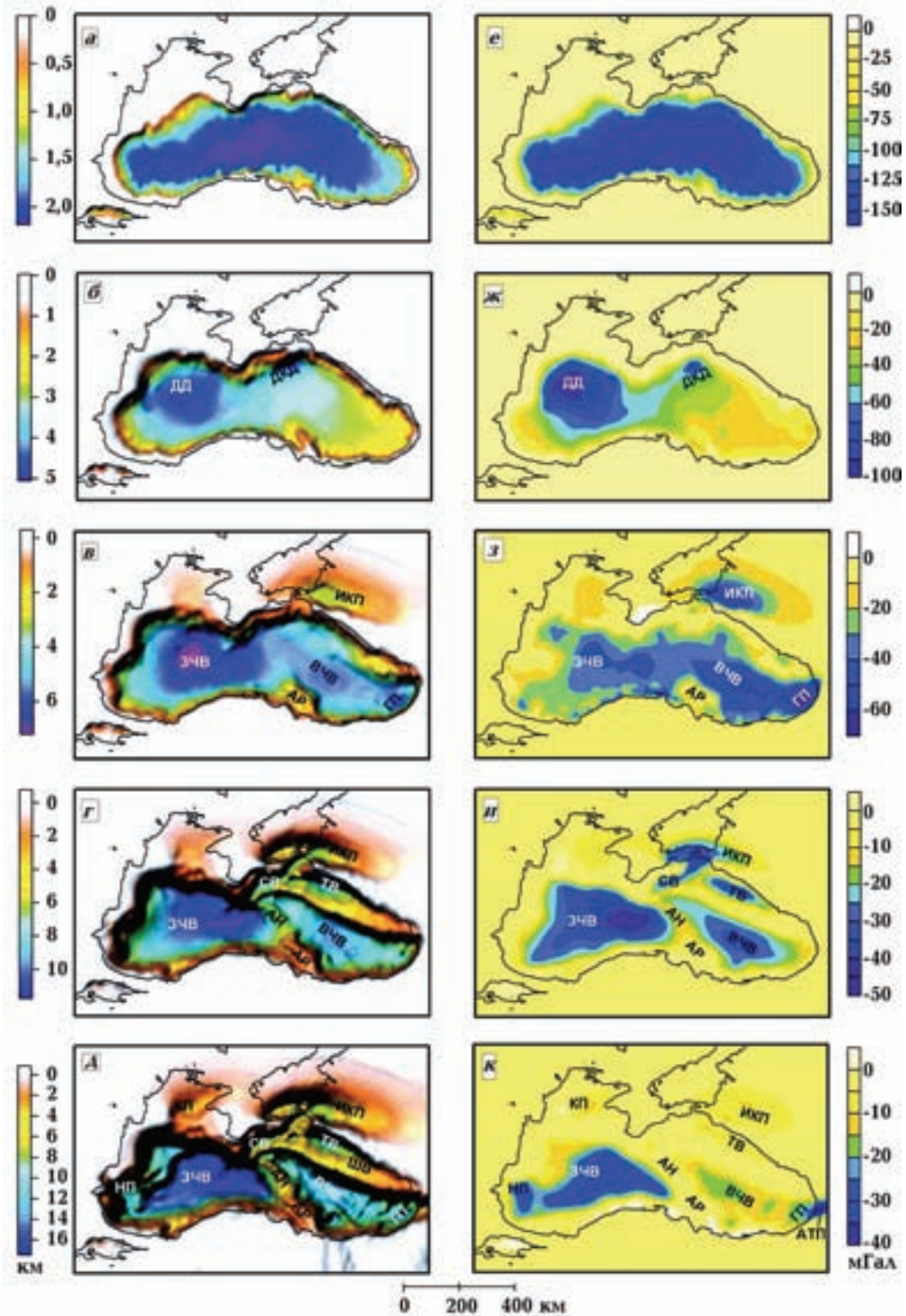
Рис. 4. Гравитационный эффект морской воды Черного моря и четырех слоев в осадках, геометрия которых задавалась по структурным картам [Туголесов и др., 1985]. Эффект слоя морской воды (e) с глубинами дна моря (a); эффект четвертичных осадков, ограниченных подошвой антропогена (б) с плотностью 2,10 \text{ г/см}^3 (ж); гравитационный эффект неогеновых осадков (плиоцен—верхне/средний миоцен) с плотностью 2,35 \text{ г/см}^3 (з) и подошвой по кровле майкопской серии (в); влияние отложений майкопской серии со средней плотностью 2,60 \text{ г/см}^3 (и), ограниченных подошвой олигоцена (г); эффект палеоцен-эоценовых пород с плотностью 2,65 \text{ г/см}^3 (к) и подошвой по кровле мела (д). АТП — Аджаро-Триалетский пояс, ГП — Гурийский прогиб, ДД — Дунайская дельта, ДКД — Доно-Кубанская дельта, КП — Каркинитский прогиб, НП — Нижнекамчийский прогиб. Остальные условные обозначения см. на рис. 2.
