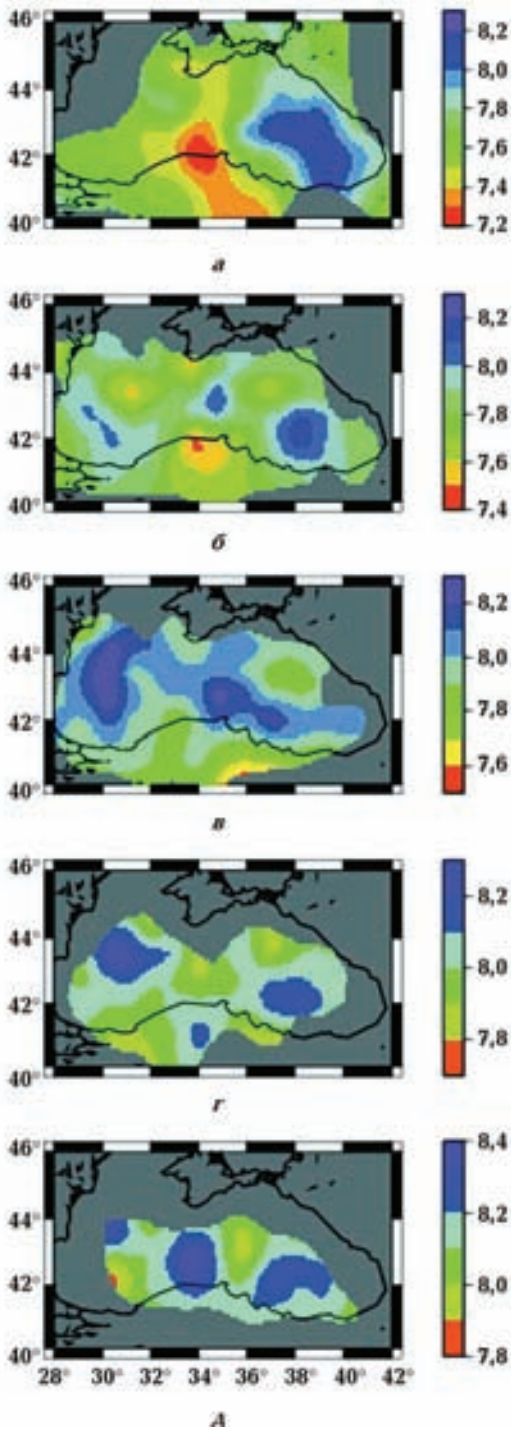
Рис. 11. P -скоростная сейсмотомографическая модель Черного моря, представлена горизонтальными сечениями скоростей для глубин 35—43 км (а), 43—50 км (б), 50—60 км (в), 60—70 км (г) и 70—85 км (д).
