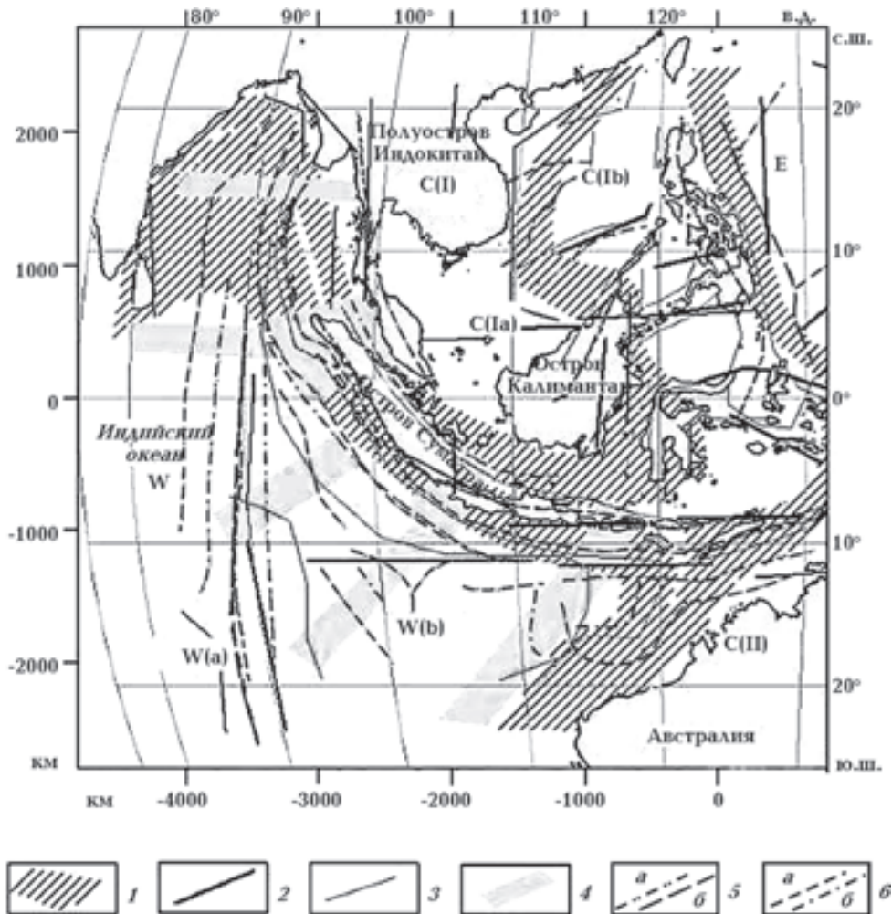
Рис. 3. Схема сегментации Зондской зоны субдукции на основе анализа гравитационного поля и дополнительной геолого-геофизической информации (по А. А. Антипову): 1—3 — градиентные зоны в полях низкочастотной компоненты гравитационного поля (1), среднечастотной компоненты (2), трансформант, рассчитанных по методу Саксова—Нигарда (3); 4 — границы сегментов, выделенных в Зондской зоне субдукции и на прилегающей к ней части Индо-Австралийской плиты; 5 — оси региональных аномалий силы тяжести по среднечастотной компоненте поля силы тяжести (а — положительных, б — отрицательных); 6 — оси положительных (а) и отрицательных (б) аномалий по высокочастотной компоненте гравитационного поля.
