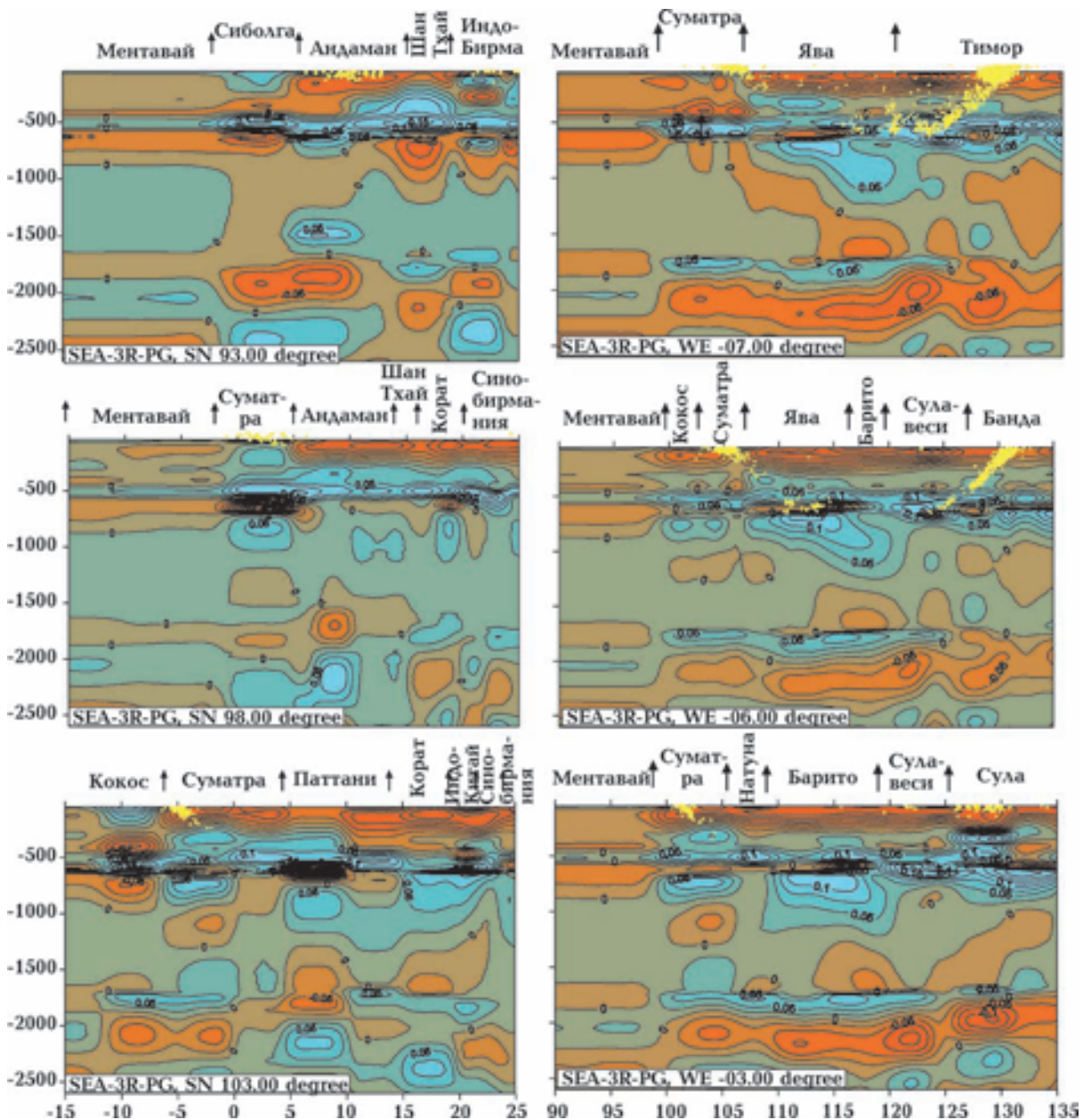
Рис. 6. Долготные и широтные сечения 3D P -скоростной модели мантии под Юго-Восточной Азией.
