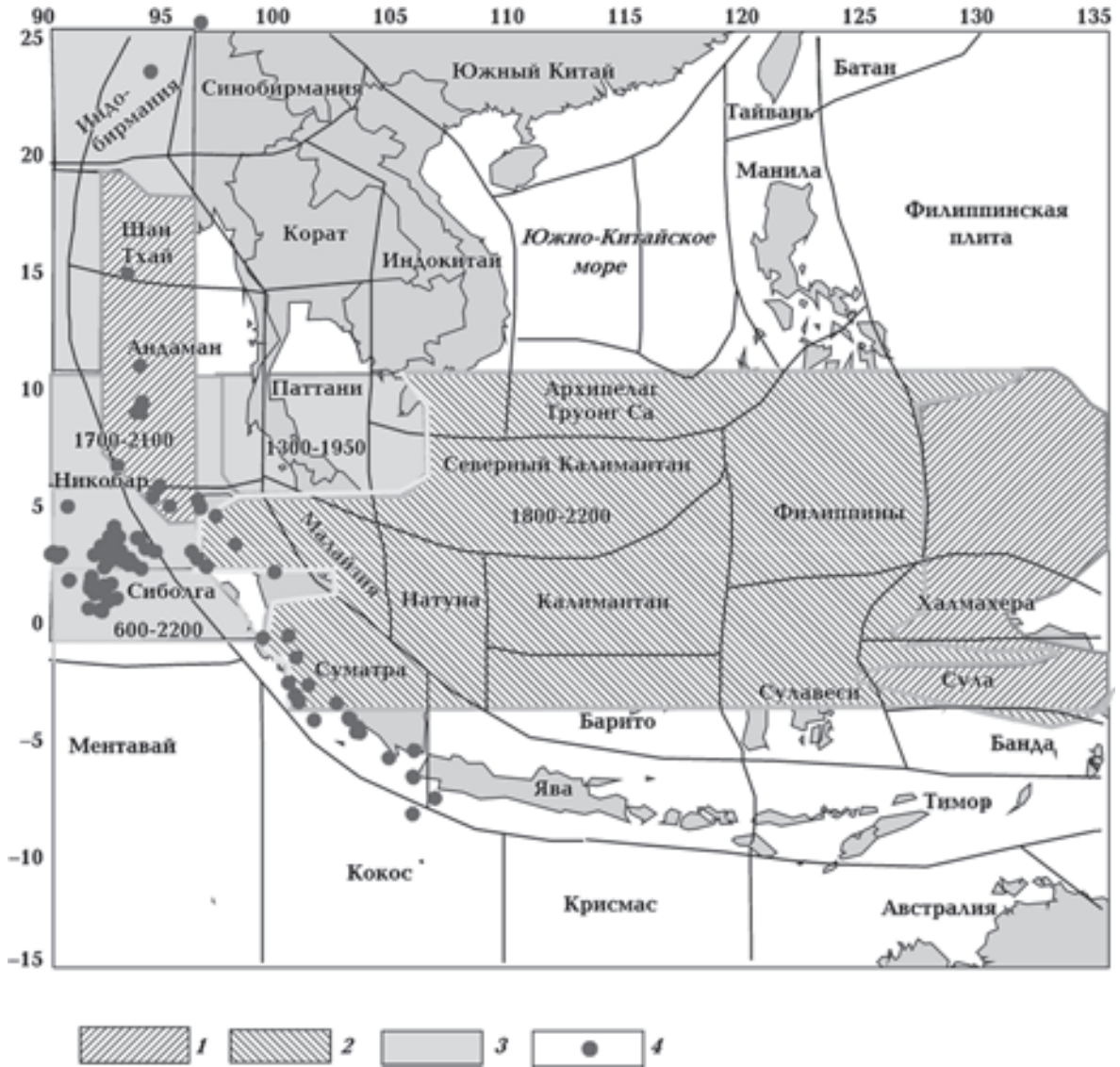
Рис. 8. Схема распространения выходов низких скоростей из нижней мантии: 1 — под Филиппинской плитой (с глубины 2600 км); 2 — под блоками Халмахера-Сула; 3 — под блоками Андаман и Шан Тхай; 4 — землетрясения за 2012 г.
