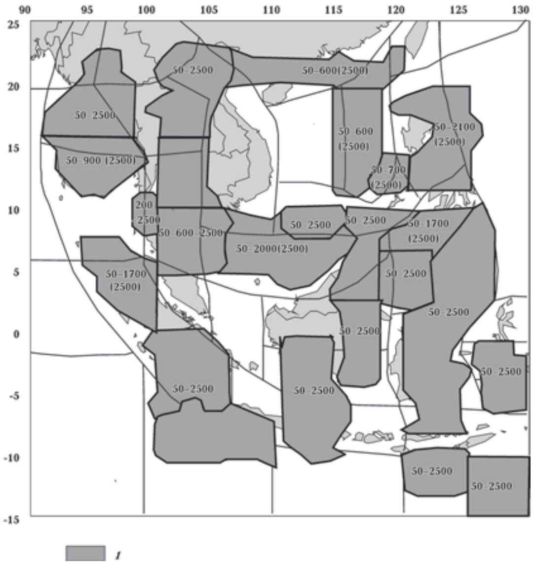
Рис. 10. Мантийные скоростные колонки, выделяемые по данным сейсмической томографии в мантии под Юго-Восточной Азией: 1 — мантийные скоростные колонки 50 км (минимальная глубина) до 2500 км (максимальная глубина).
