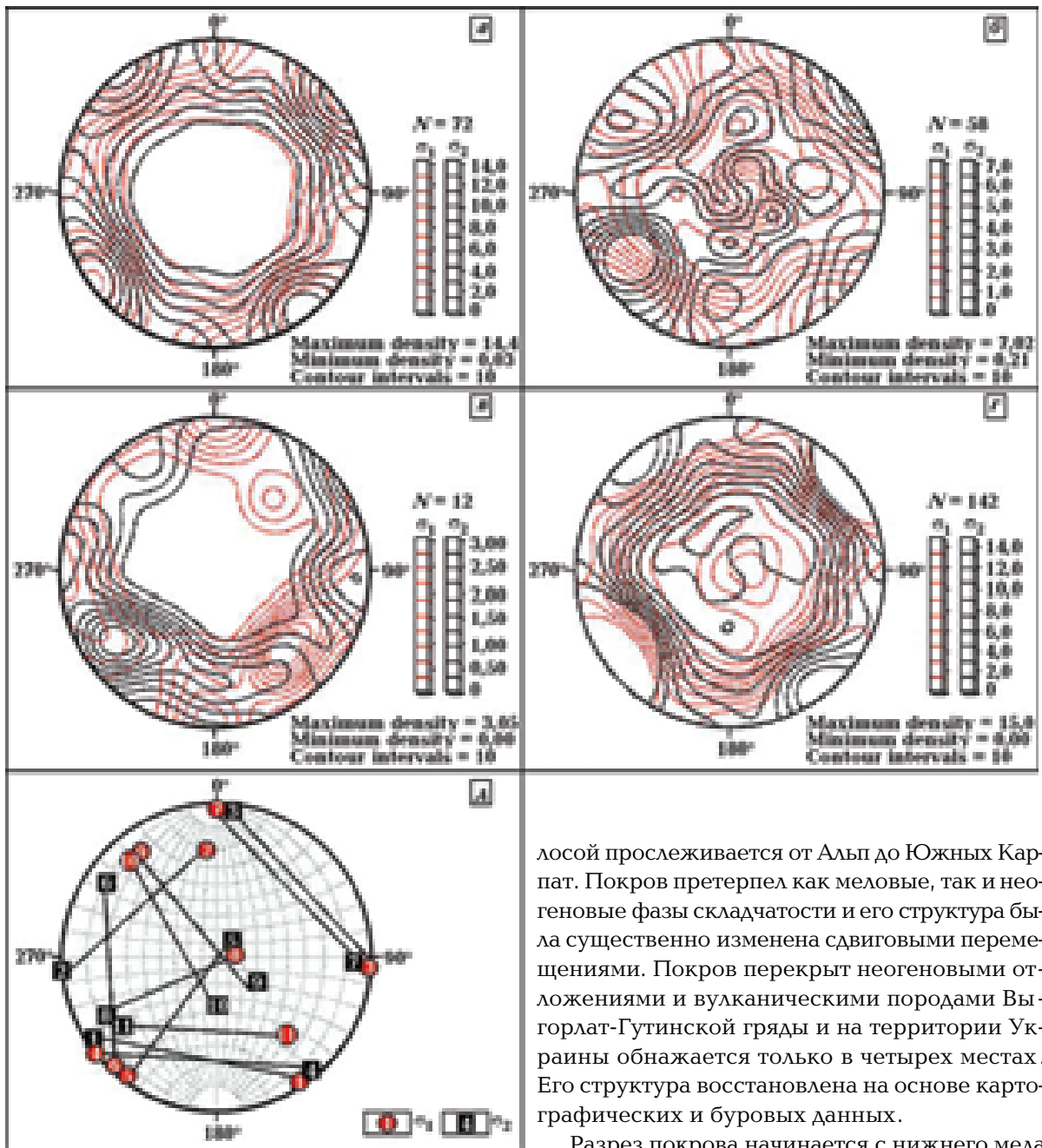
Рис. 7. Стереогаммы изолиний концентрации осей сжатия ( \sigma_1 ) и растяжения ( \sigma_3 ), построенные с помощью программы Stereo 32. Цифры в квадратах и кружках на рис. 7, д соответствуют номерам полей в табл. 3. Остальные пояснения в тексте.
