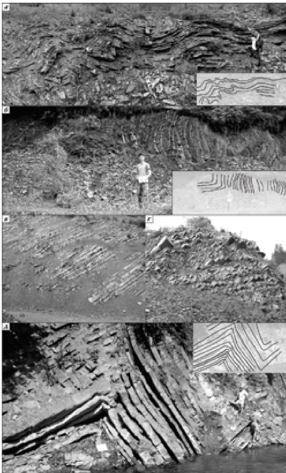
Рис. 3 Деформации пород флишевой толщи УК вдоль профиля РАНСАКЕ: а, б — деформации тонкослойной песчано-глинистой толщи (с преобладанием глинистой составляющей) в верховинской свите. Кросненский покров, точки наблюдений 12, 16; в, г — моноклинальное залегание эоценовых песчаников. Скибовый покров. Точки наблюдений 30, 31; д — шевронные подобные складки, нарушенные в замках разрывами. Скибовый покров, стрыйская свита.
