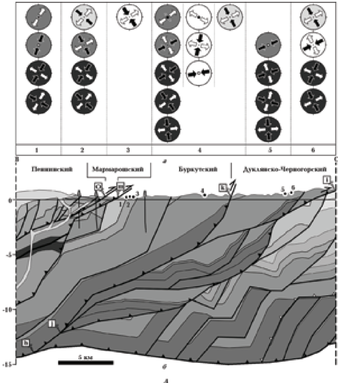
Рис. 6. Результаты тектонофизических исследований вдоль профиля PANCAKE: А — Пеннинский, Мармарошский, Буркутский и Дуклянско-Черногорский покровы; Б — Кросненский покров; В — Скибовый покров. Стереогаммы осей напряжений (а) над сбалансированным геоло-
