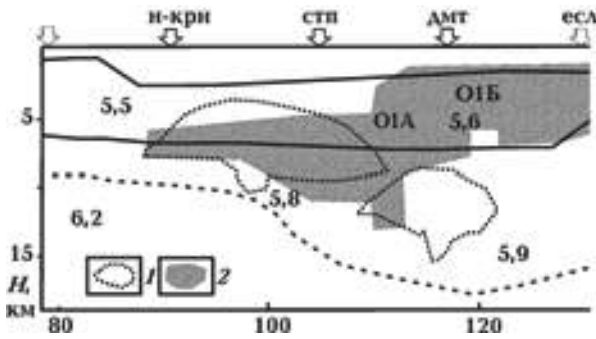
Рис. 6. Геологический разрез зоны магматической активизации в районе Амвросиевского купола, совмещенный с линией сейсмического профиля ГСЗ XI [Александров и др., 1996]: 1 — контуры предполагаемых интрузивных тел, 2 — ОПС О1 со значениями \rho < 20 \text{ Ом} \cdot \text{м} . Остальные обозначения см. на рис. 5.
