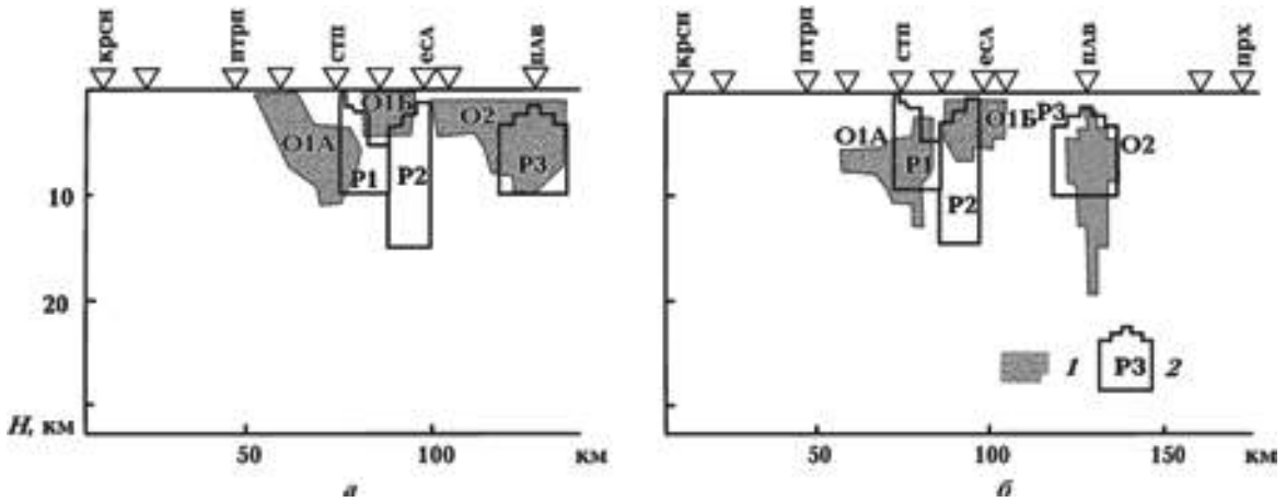
Рис. 4. Сопоставление результатов 2D моделирования по инверсии (1) и прямой (2) задаче для моделей: а — te_m10, б — te-tr-tm_m03. Аббревиатура О1—О2 соответствует результатам настоящей работы, а Р1—Р3 — работе [Рокитянский и др., 1994].
