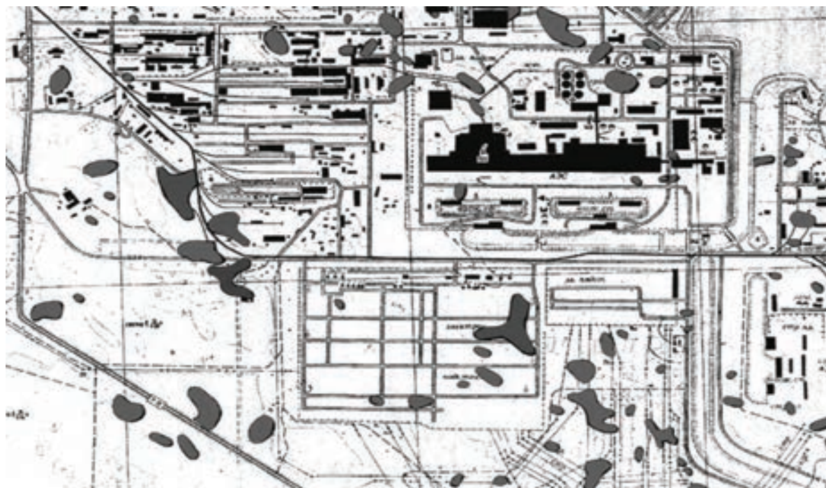
Рис. 7. Активные западины на площадке ЧАЭС (обозначены серыми пятнами).
