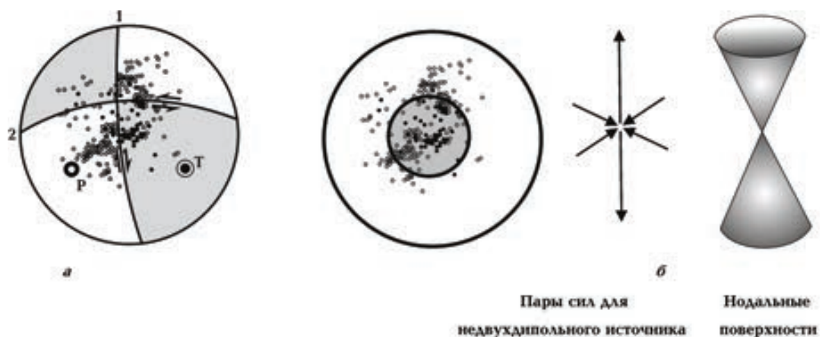
Рис. 7. Осредненный механизм для области 3(3) для двухдипольного (а) и недвухдипольного (б) источника. Условные обозначения см. на рис. 3.
