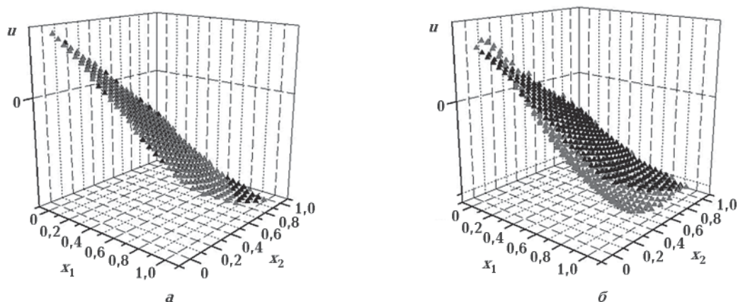
Результаты решения задачи (18) с помощью модифицированного аддитивно-усредненного расщепления и схемы явного счета (серый — численное решение, черный — аналитическое): а — \tau = 0,01, m = 1 ; б — \tau = 0,1, m = 10 .
