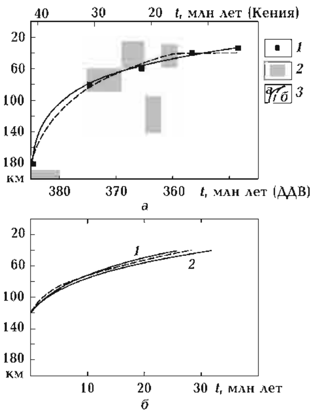
Рис. 1. Тестирование предлагаемого подхода для исходной литосферы мощностью 185 км; 1—2 — данные о глубине и времени формирования магм в Кенийском (1) и Днепровско-Донецком (2) рифтах (по [Wendlandt, Morgan, 1982; Усенко, 2004]); 3 — теоретическая кривая подъема границы литосфера/астеносфера для Кенийского рифта (а) [Mogeschal, Gliko, 1991] и траектория подъема границы, полученная с помощью используемой модели (б) и сравнение результатов расчета термального утонения литосферы мощностью 120 км из работ [Crough, Thompson, 1976] (1), [Зорин, Лепина, 1984] (2) и используемой модели (3) (б).
