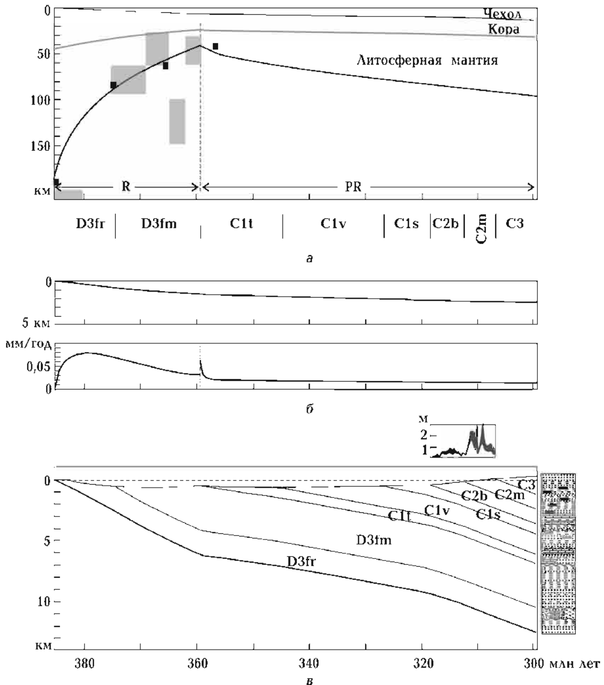
Рис. 10. Модель погружения осевой зоны юго-восточной части ДДВ: а — эволюции литосферы (показаны положения очагов магмы при формировании рифтов Восточной Африки и ДДВ, по [Wendlandt, Morgan, 1982; Усенко, 2004] (см. рис. 1, а)); кривые тектонического погружения (вверху) и его скорости (б) и осадконакопление (в) (вверху — график изменения средней мощности угольных пластов во времени для паралической угленосной формации Донбасса [Феофилова, Левенштейн, 1963]).
