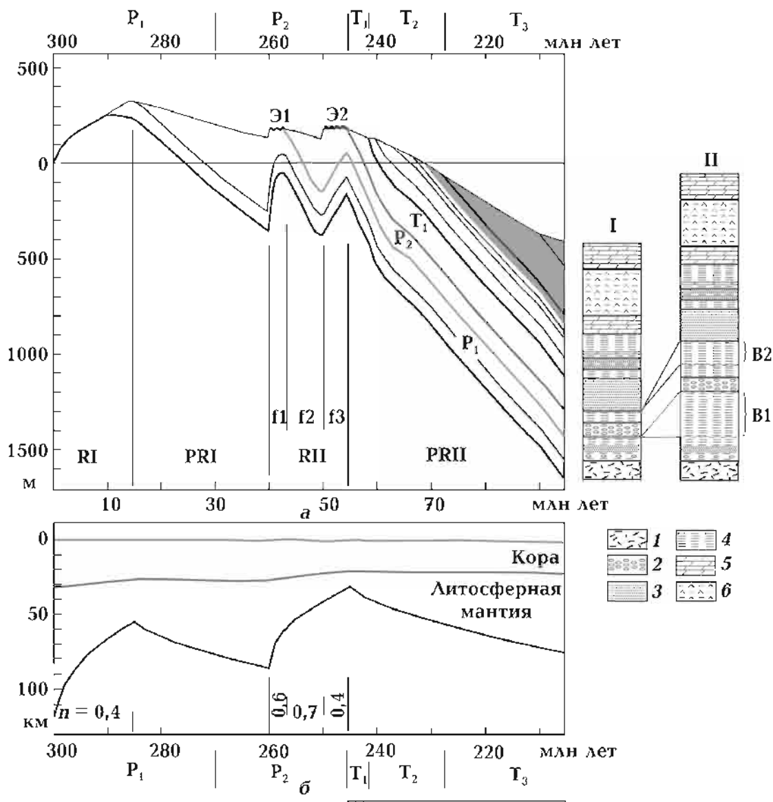
Рис. 6. Пример моделирования погружения осадочного бассейна Эбро (Иберия): а — модель вертикальных движений фундамента и осадконакопления; RI, RII — этапы активного рифтогенеза; PRI, PRII — пострифтового погружения, f1, f2, f3 — фазы рифтинга; Э1, Э2 — эрозионные события; морская часть модельного разреза тонирована (I — наблюдаемый осадочный разрез северо-западной части впадины Эбро (по [Vargas et al., 2009]), II — тоже, но с восстановленными эродированными отложениями (B1, B2); 1 — вулканиты, 2 — конгломераты, 3 — песчаники, 4 — глины, 5 — доломиты, 6 — эвапориты); б — смещение границ литосферы в модели; для этапов рифтогенеза показаны принятые величины индекса утонения коры n ; в — диаграмма скоростей осадконакопления для триасовой части моделируемого разреза; оцифрованные кривые — теоретическая скорость компенсированного осадконакопления в условиях пострифтового остывания литосферы [Гончар, 2013].
