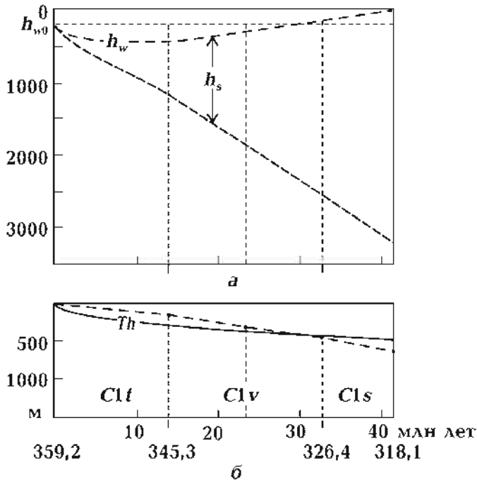
Рис. 9. Пример расчета погружений фундамента и морских глубин депоцентра юго-восточной части ДДВ в раннем карбоне (а) и траектории термального погружения в модели ( th ) и реконструированного тектонического методом бэкстриппинга без учета морских глубин (пунктир) (б). См. пояснения в тексте.
