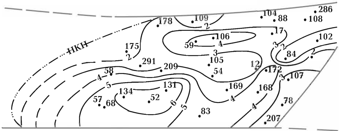
Рис. 4. Карта распределения неоднородности по проницаемости ( K_{пр}/(P \cdot И) ) по SP_v месторождения Гюнешли (VII блок).
