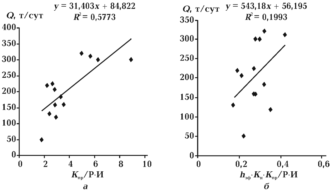
Рис. 2. Зависимости начальных дебитов скважин от параметров неоднородности: а — K_{пр}/(P \cdot I) , б — (h_{эф} \cdot K_n \cdot K_{пр})/(P \cdot I) .
