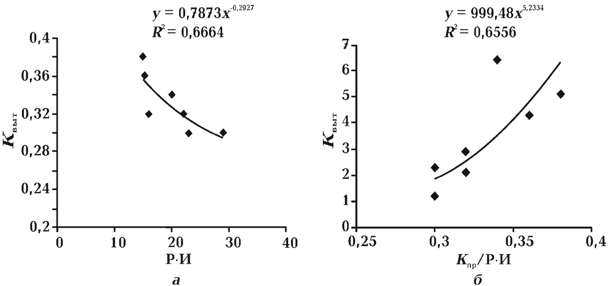
Рис. 3. Зависимости коэффициента вытеснения нефти от параметров неоднородности пласта-коллектора (СПв): а — P \cdot I , б — K_{пр}/P \cdot I .
