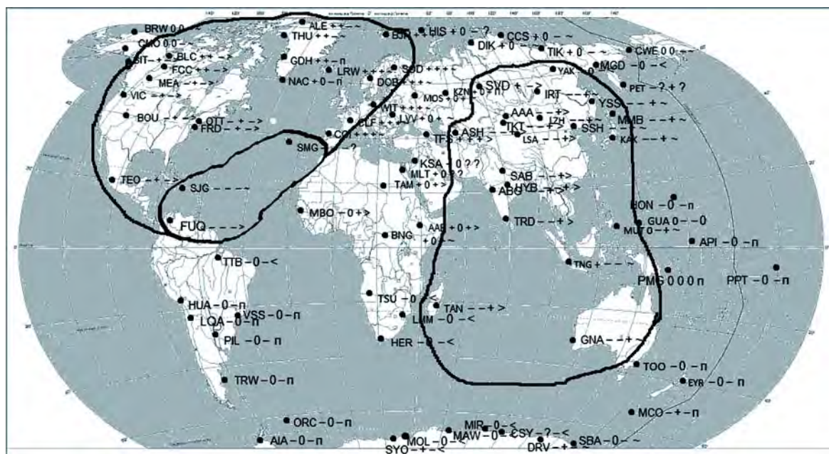
Рис. 9. Карта змін знака BB(T) на обсерваторіях світової сітки у 19—24-му циклах сонячної активності. Позначення: "+" — напруженість поля зростає при BB(T) > 0 або спадає сповільнюється при BB(T) < 0 ; "-" — напруженість поля спадає при BB(T) > 0 або зростає при BB(T) < 0 ; ">" — BB(T) збільшується за абсолютною величиною після 21-го циклу; "<" — BB(T) зменшується за абсолютною величиною після 21-го циклу; "n" — BB(T) не змінюється за абсолютною величиною після 21-го циклу; "-?" — BB(T) змінюється за абсолютною величиною; "?" — даних BB(T) немає; "0" — ефект 20-го циклу не спостерігається.
