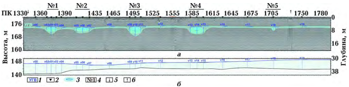
Рис. 15. Вертикальный разрез зон повышенного увлажнения почв на участке строительства, ограждающей конструкции заглубленных сооружений (по геофизическим данным на 27—30 июля 2017 г.): а — вертикальный разрез зон повышенной фильтрации грунтовых вод в верхней части строительства ограждающих конструкций; б — вертикальный разрез зоны увлажнения песков полтавской свиты (нижний водяной горизонт): 1 — уровень грунтовых вод по состоянию на 28.07.2017; 2 — пункты ВЭРЗ (V00—V19); 3 — зоны повышенной фильтрации грунтовых вод ("подземные водяные потоки"); 4 — номер водного потока; 5 — начало зоны закрепления; 6 — угол забора.
