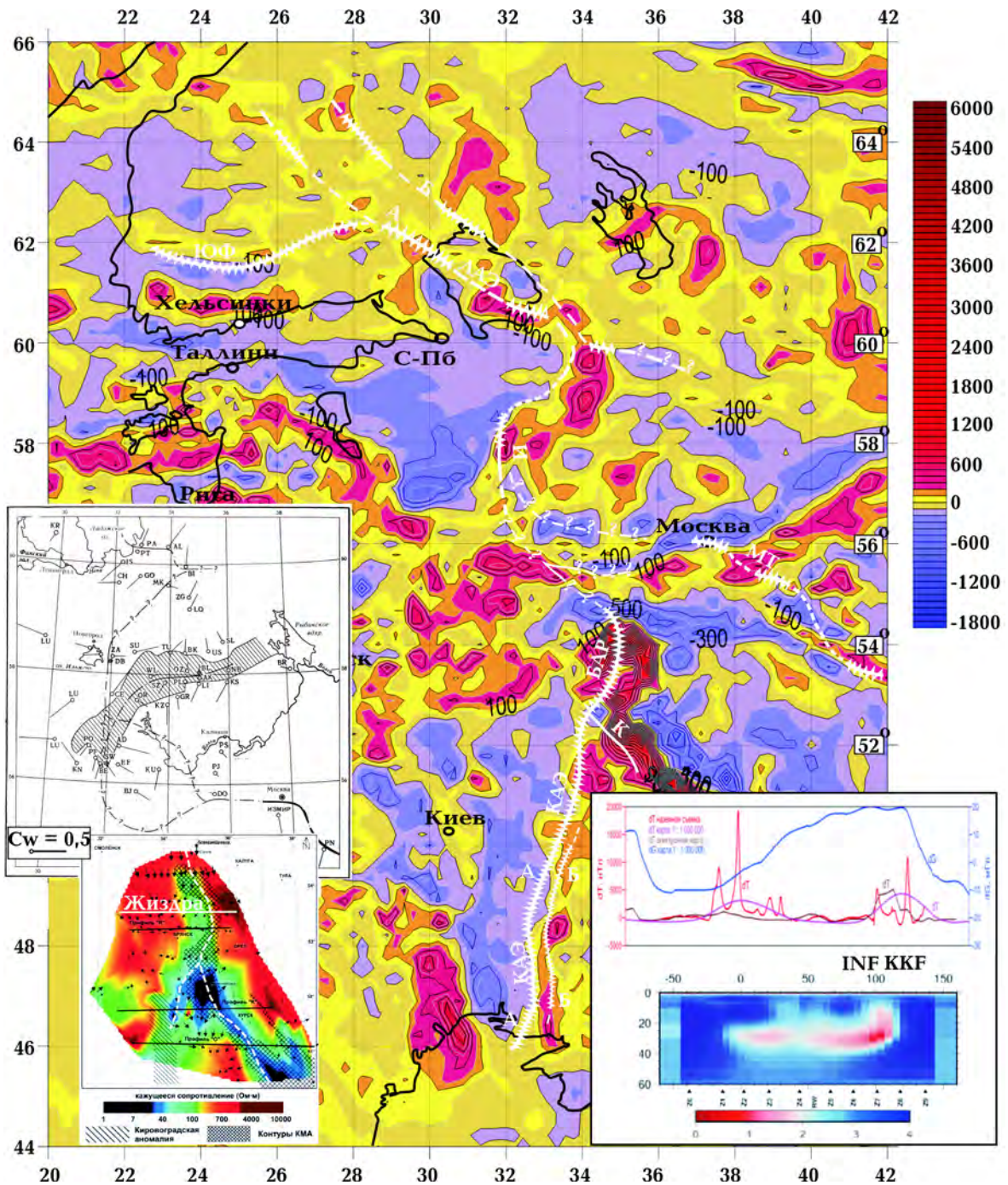
Рис. 12. Трансъевропейская цепь аномалий электропроводности (ТЕЦАЭ) (дана белым цветом): Кировоградская (КАЭ, проводники А и Б), Барятинская (БАР с ответвлением К — Курская аномалия), Ладожско-Ильменская (ЛАЭ + И), Московско-Тамбовская (МТ) и Южно-Финляндская (ЮФ) представлены на фоне карты аномалий постоянного магнитного поля. На врезке слева даны карты векторов индукции (верхняя из работы [Рокитянский и др., 1982, рис. 1] представляет векторы Визе, полученные по вариациям с периодом от 10 до 60 мс., заштрихованная полоса — Валдайский грабен; нижняя левая врезка из работы [Куликов и др., 2018, рис. 3], на ней даны действительные векторы для периода 300 с на фоне изолиний эффективного кажущегося сопротивления на периоде 300 с). Белый пунктир показывает ось Барятинской аномалии, которая южнее 53° с. ш. раздваивается на две ветви: западная соединяется с КАЭ, а восточная, названная Курской (К) аномалией, уходит на юг—юго-восток. Белый отрезок показывает профиль “Жиздра”. Врезка справа из работы [Алексанова и др., 2011, рис. 3];
