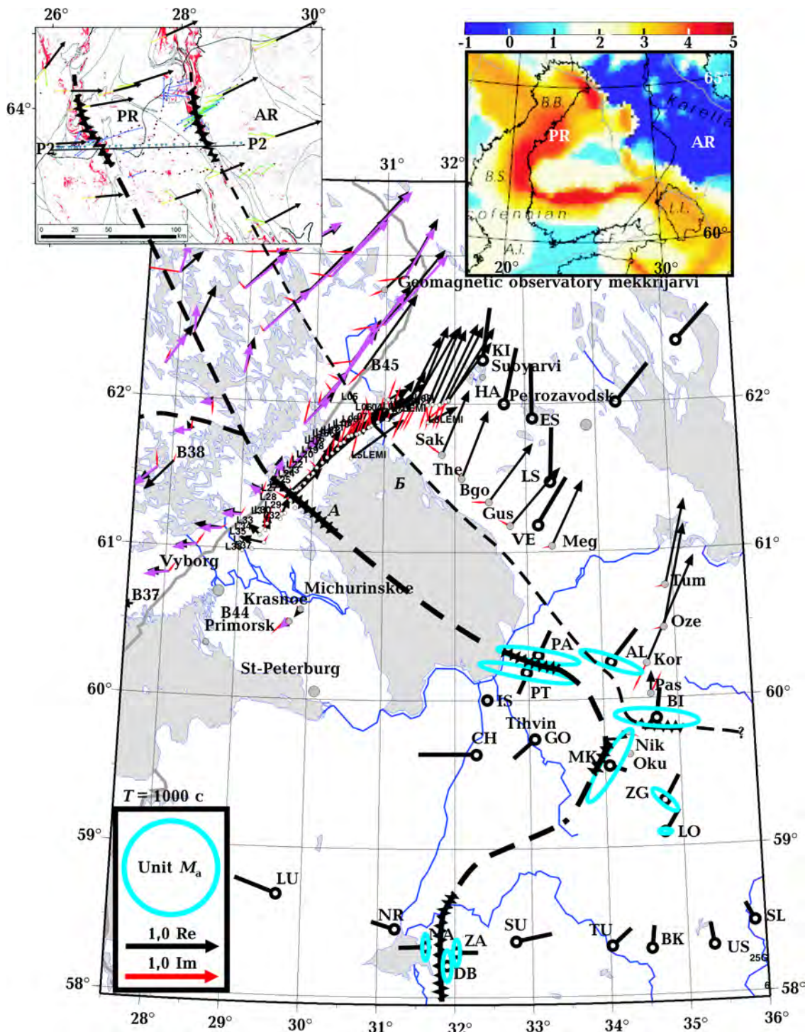
Рис. 10. Гипотезы продолжения ЛАЭ в северо-западном, юго-восточном и южном направлениях.
