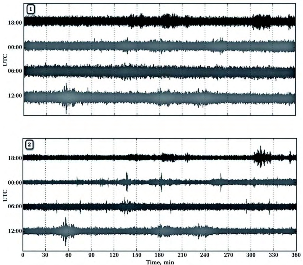
Рис. 1. 24-годинна графічна реалізація цифрового сейсмонахиломірного запису з 18:00 22.03.17 по 18:00 23.03.17 (UTC) під час вибухів у Балаклії: 1 — чотири 6-годинні інтервали нефільтрованих цифрових записів; 2 — ті самі записи після цифрової смугової фільтрації (1—3 Гц). Масштаби: по вертикалі — сейсмічні сигнали, мВ; по горизонталі — час, хв.
