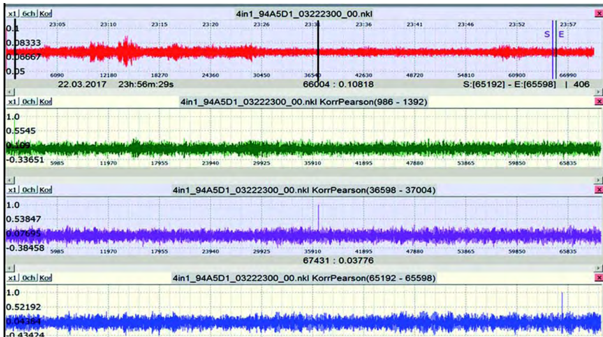
Рис. 4. Балаклія, 23:00 (UTC) 22 березня. Запис сейсміки до і після початку вибухів (вверху) та 3 корелограми (внизу) за відсутності сейсмопакетів (тут і надалі початок кожного тест-інтервалу, тобто "корелятора", позначено вертикальними лініями).
