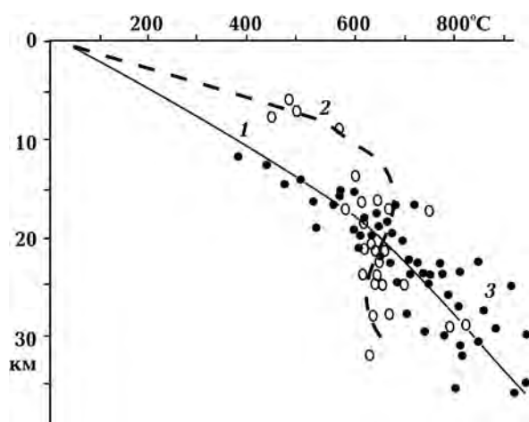
PT -условия регионального метаморфизма в коре УЩ (1), распределение температур при гидротермальной активности (2), PT -условия метаморфических и гидротермальных преобразований, установленные для метаморфических пород УЩ (точки 3) (по работе [Гордиенко, 2007]).
