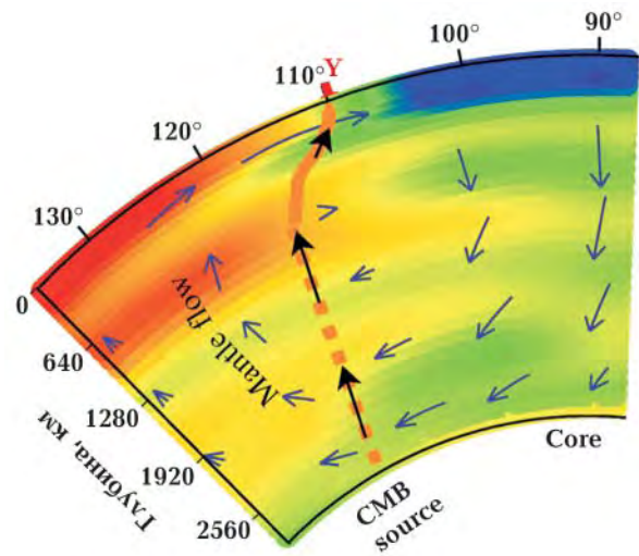
Рис. 3. Пересечение Йеллоустонского плюма с конвекционной ячейкой S-волны [Smith et al., 2009]. Для построения скоростного сечения S-волн мантии в западной части Северной Америки использована работа [Su et al., 1994]. Направления и скорость мантийного потока представлены векторами. Холодные цвета — относительно высокие, а теплые цвета — относительно низкие скорости.
