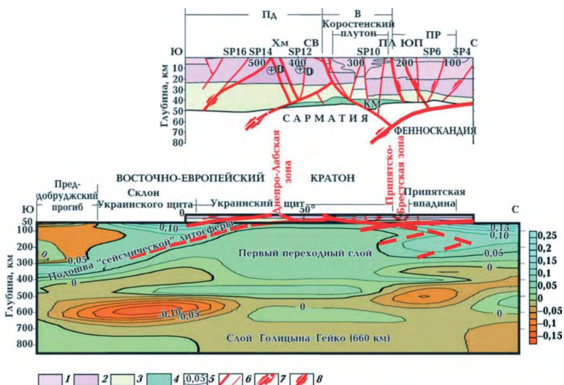
Рис. 10. Тектоническая интерпретация данных ГСЗ, плотностной модели и сейсмотомографии вдоль геотраверса Евробридж-97 [Bogdanova et al., 2006]: 1—4 — петрофизические слои консолидированной земной коры (1 — «гранитный», 2 — «диоритовый», 3 — «базальтовый», 4 — «коромантийная смесь»); 5 — изолинии \Delta V_p ; 6 — зоны разломов, сопровождавшие субдукционный процесс (слева) и разломы высших порядков; 7 — левый сдвиг; 8 — правый сдвиг.
