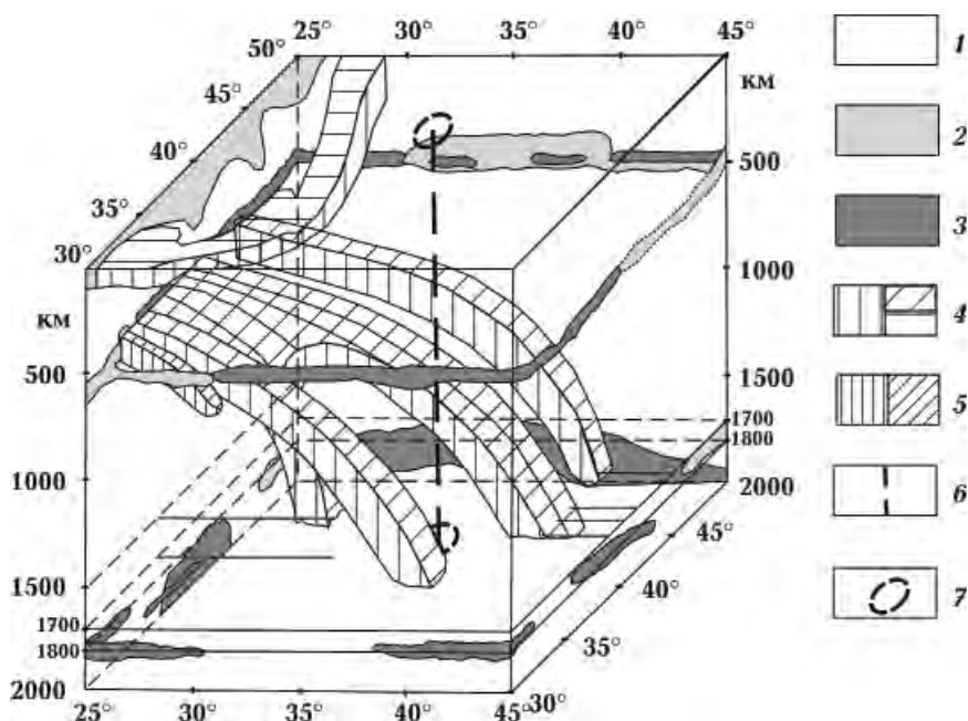
Рис. 2. Блок-диаграмма района исследований, отображающая соотношения верхнемантийных встречных слэбов и среднемантийных наклонных даунвеллингов [Гинтов и др., 2016]: 1 — вмещающая, главным образом относительно низкоскоростная (по значениям невязок \Delta V_p км/с) среда в мантии; 2 — относительно низкоскоростные неоднородности ( \Delta V_p \leq 0,15 км/с); 3 — относительно высокоскоростные, в основном широтно вытянутые неоднородности ( \Delta V_p \geq 0,025 км/с); 4 — штриховка поверхностей относительно высокоскоростных слэбов и даунвеллингов: вертикальная — боковые, косая и горизонтальная — верхние; 5 — то же относительно низкоскоростных даунвеллингов; 6 — вертикальная ось мантийной колонки (плюма); 7 — следы пересечения колонки с подошвами верхней и средней мантии (в данной работе мантийная колонка не рассматривается).
