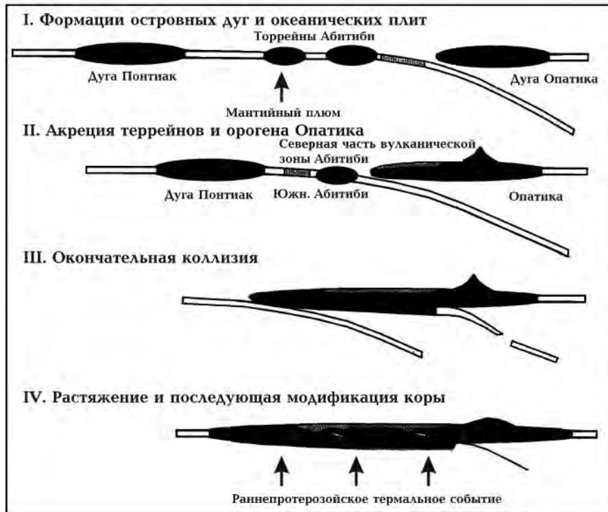
Рис. 4. Схема процесса формирования архейской коры северо-восточной части провинции Сьюперитор, по [Calvert, Ludden, 1999]. Зоны субдукции идентифицированы по нескольким сейсмическим профилям через пояса Опатика, Абитибби и Понтиак. Наличие коматиитов на юге Абитибби указывает на вероятное взаимодействие океанической коры с одним или несколькими мантийными плюмами.
