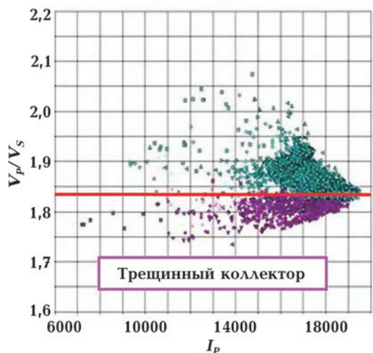
Рис. 11. Кросс-плот отношения скоростей V_P/V_S и акустического импеданса I_P , измеренного в (м/с) ( \text{г/см}^3 ), для силурийского карбонатного резервуара в Тимано-Печорской провинции с выделением двух литотипов, которые хорошо разделяются красной линией [Федотов и др., 2009].
