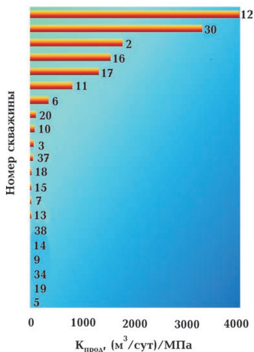
Рис. 16. Среднеарифметические значения коэффициентов продуктивности скважин (сверху вниз по мере уменьшения) [Хромова, 2008].
