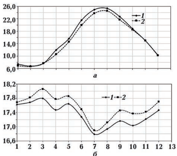
Рис. 2. Сезонный ход осредненных по широте за 1998—2000 гг. среднемесячных значений температуры (а) и солености (б) поверхностного слоя воды на черноморском шельфе (кривая 1) и в проливе Босфор (кривая 2).
