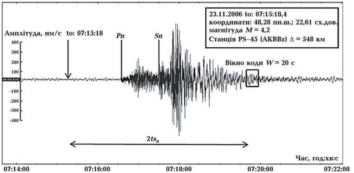
Рис. 1. Вихідний (нефільтрований) запис землетрусу 23 листопада 2006 р. (час уджерелі: t_0 = 07:15:18,4 ; магнітуда M = 4,2 ), отриманий на станції PS-45AKBBz, \Delta = 548 км (м. Малин).
