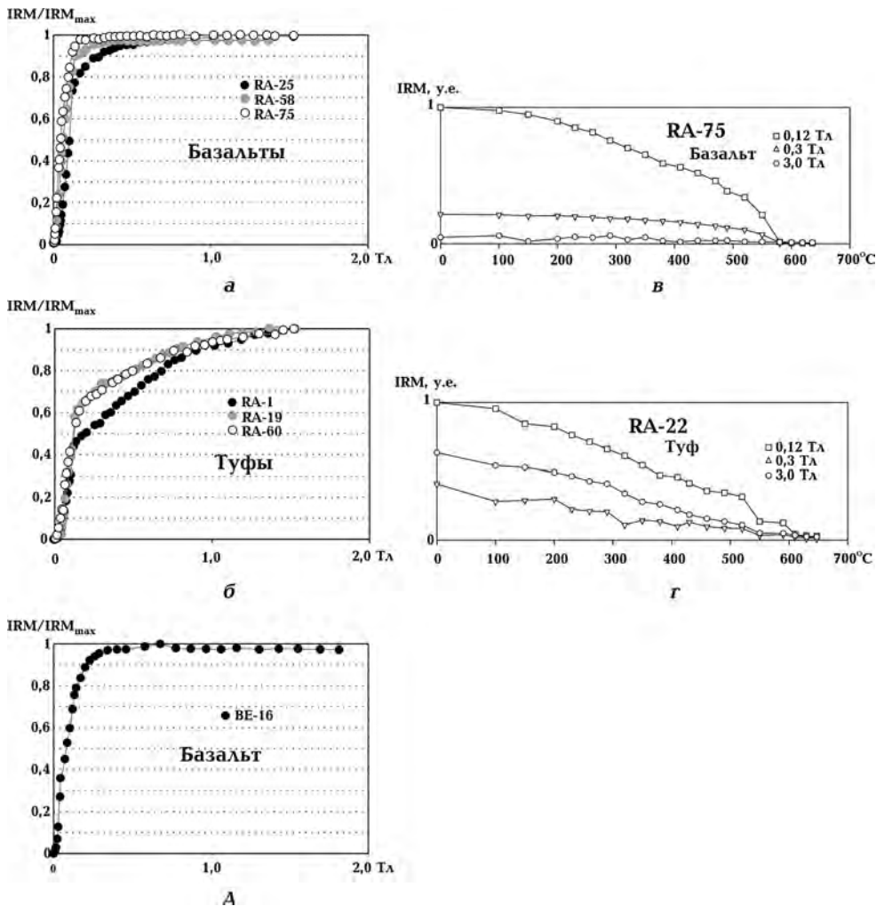
Рис. 10. Кривые ступенчатого изотермического намагничивания (IRM) образцов базальтов и туфов карьеров Рафаловка (а, б), Берестовец (v) и кривые терморазмагничивания наведенной вдоль трех ортогональных осей IRM в полях 3,0, 0,3 и 0,12 Тл (B, Г).
