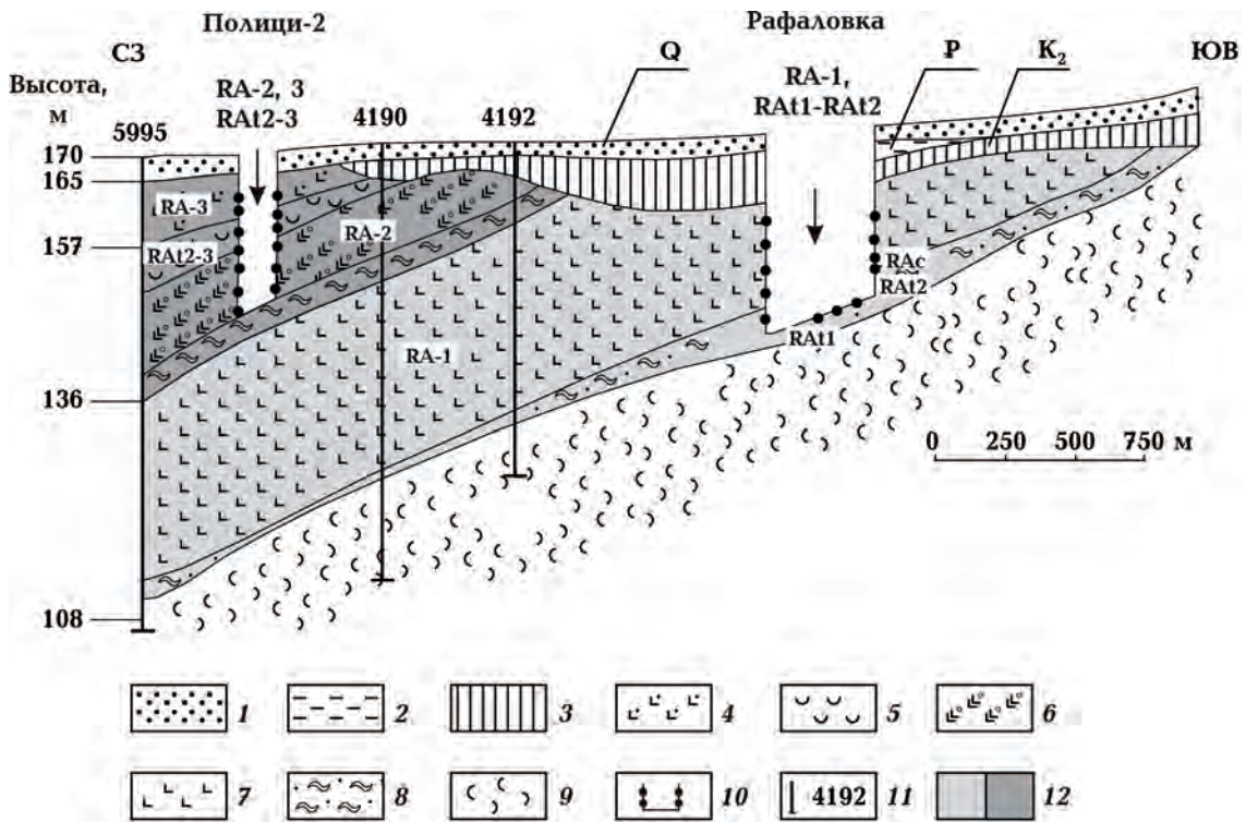
Рис. 2. Стратиграфическое соотношение трапových толщ карьеров Полици-2 и Рафаловка (схема модифицирована из работы [Глеваская и др., 2006]): 1—3 периоды (1 — Q; 2 — P; 3 — K 2 ); 4 — третий базальтовый поток RA-3; 5 — туфы RA2-3; 6 — второй базальтовый поток RA-2; 7 — первый базальтовый поток RA-1; 8 — туфы RA1-1, RA1-2; 9 — лавобрекции; 10 — места отбора образцов; 11 — скважины; 12 — антиподальная полярность.
