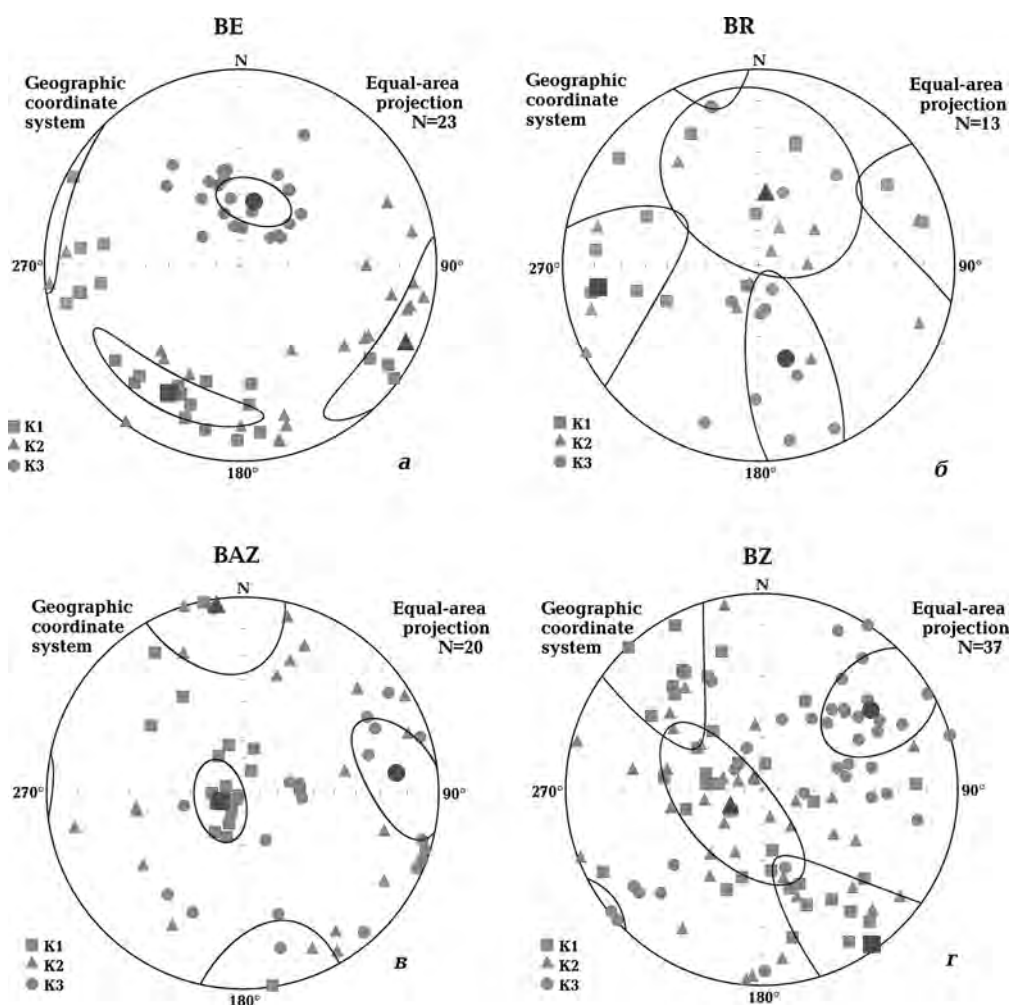
Рис. 9. Стереографические проекции направлений осей эллипсоида АМВ образцов карьеров Берестовец (BE, BR) и Базальтовое (BAZ, BZ) в географической системе координат. Условные обозначения см. на рис. 6.
