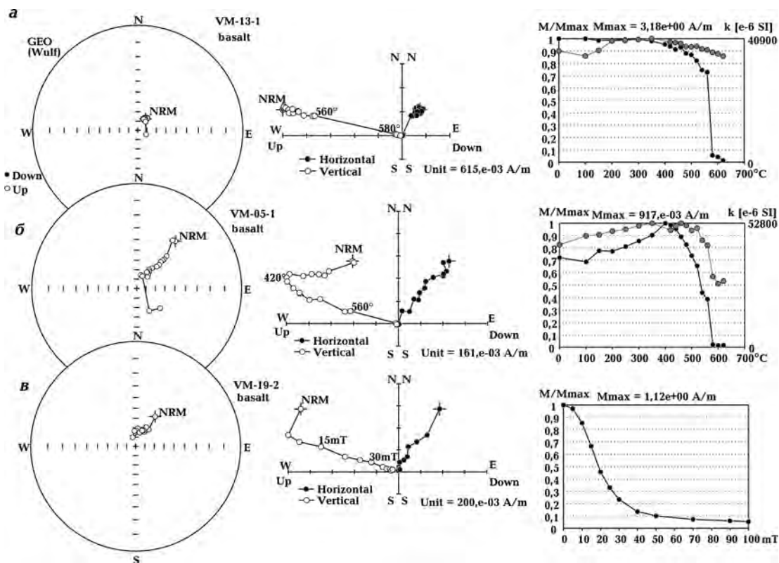
Рис. 7. Результаты ступенчатого терморазмагничивания (а, б) и размагничивания переменным магнитным полем (в) образцов базальтов из карьера Великий Мидск. Условные обозначения см. на рис. 4.
