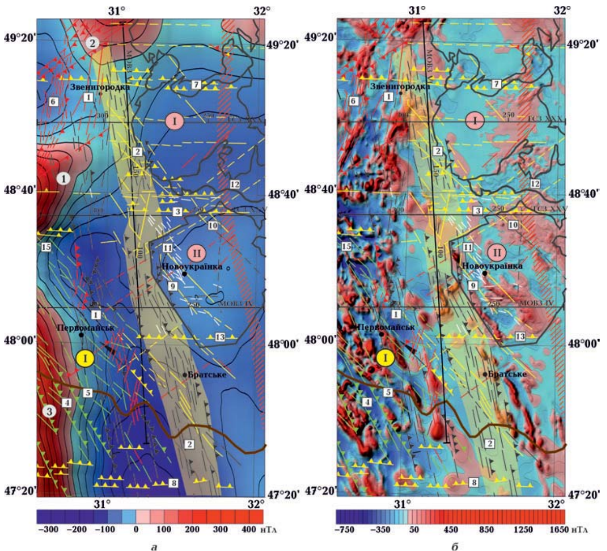
Рис. 2. Карти компонент аномального магнітного поля: регіональної (\Delta B)_{\text{а.рег.}} (а), локальної (\Delta B)_{\text{а.лок.}} (б), локальної «середньохвильової» (\Delta B)_{\text{а.лок.сх.}} (в), локальної «короткохвильової» (\Delta B)_{\text{а.лок.кх.}} (г). Регіональні магнітні аномалії (цифри в кружках): 1 — Київська, 2 — Гайсинська, 3 — Ананіївська. Пунктирні чорні лінії — осі магнітних аномалій. Інші умовні позначення див. на рис. 1.
