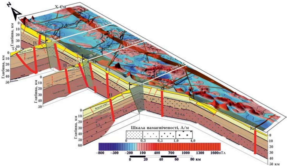
Рис. 4. Блок-схема глибинної будови Звенигородсько-Братської зони розломів за результатами магнітного моделювання вздовж профілів ГСЗ ХХХ, ХХV та МОВЗ ІV, ІVІ (складено з використанням праць [Крюченко, 1987, Ильченко, 2003; Куприенко и др., 2007; Макаренко та ін., 2021]). Скорочення: Х-См — трансрегіональний тектонічний шов Херсон—Смоленськ, зони розломів: Тл — Тальнівська, З-Б — Звенигородсько-Братська, НУ — Новоукраїнська, С-М — Суботсько-Мошоринська, Гл — Глодоська, П — Первомайська.
