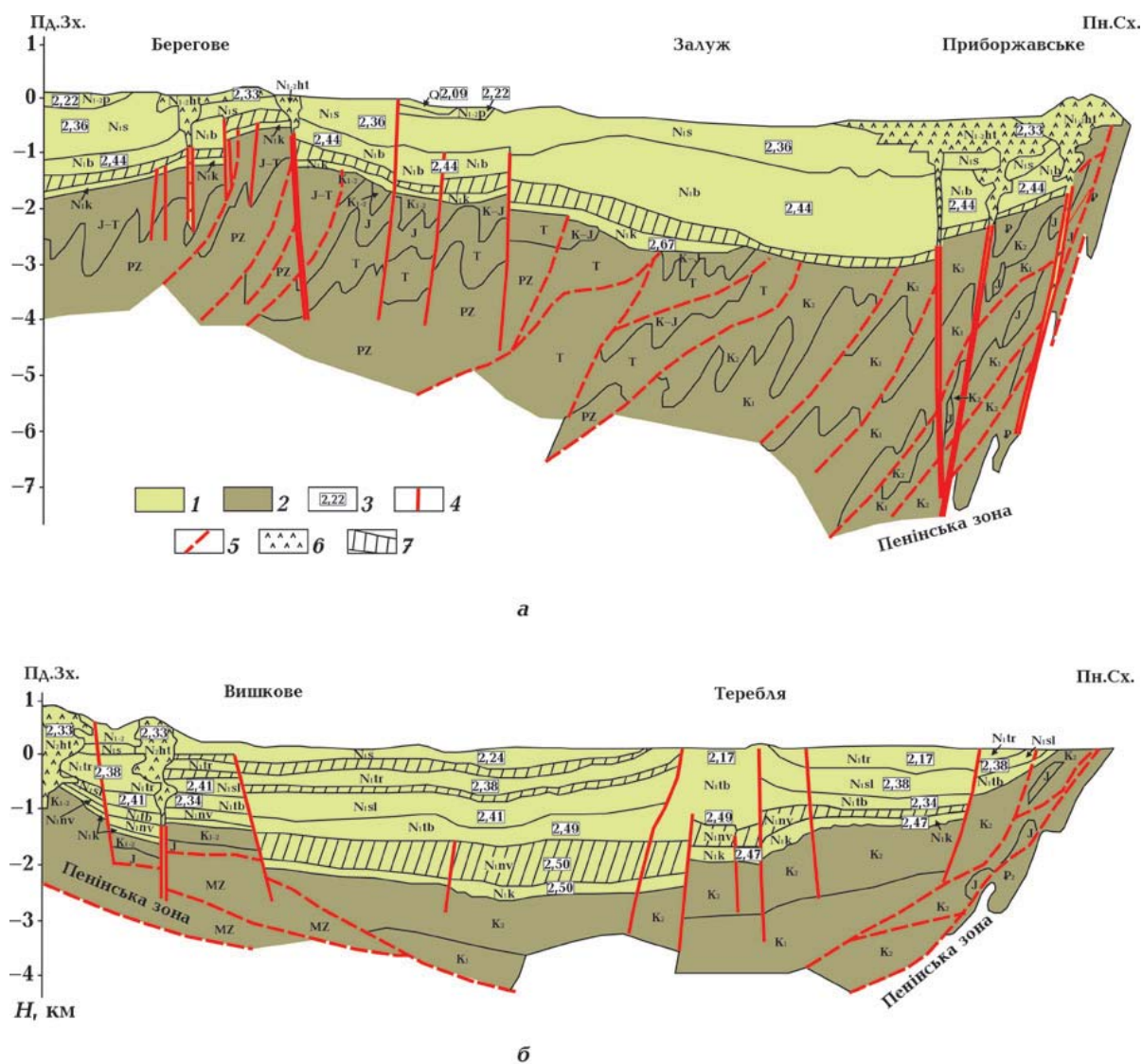
Рис. 5. Геологічні розрізи 1—1 через Мукачівську западину за лінією Берегове—Залуж-Приборжавське (а) та 2—2 через Солотвинську западину за лінією Вишкове—Теребля (б) за [Лозиняк, Місюра, 2010] зі спрощеннями: 1 — відклади верхнього структурного поверху: Q — четвертинні; неогенові : N_{2cp} — чопської світи, N_{2ht} — гутинської світи, N_{1-2p} — паннонського ярусу, N_{1s} — сарматського ярусу, N_{1b} — баденського ярусу ( N_{1tr} — тересвинської світи, N_{1sl} — солотвинської, N_{1tb} — тереблінської, N_{1lv} — новоселицької світи), N_{1k} — карпатського ярусу; 2 — відклади нижнього структурного поверху (фундаменту): P — палеоген; MZ — мезозой: K_2 — верхня крейда, K_{1-2} — нижня та верхня крейда, K_1 — нижня крейда, K—J — юра та крейда, J — юра, J—T — юра та триас, T — триас; PZ — палеозой; 3 — середнє значення густини, за [Субботин, 1955; Бородатый и др., 1965; Хоменко, 1971; Биличенко и др., 1972; Макаренко, 2021]; 4 — розломи; 5 — насуви; 6 — інтрузивні породи; 7 — туфи. Положення профілів див. на рис. 1.
