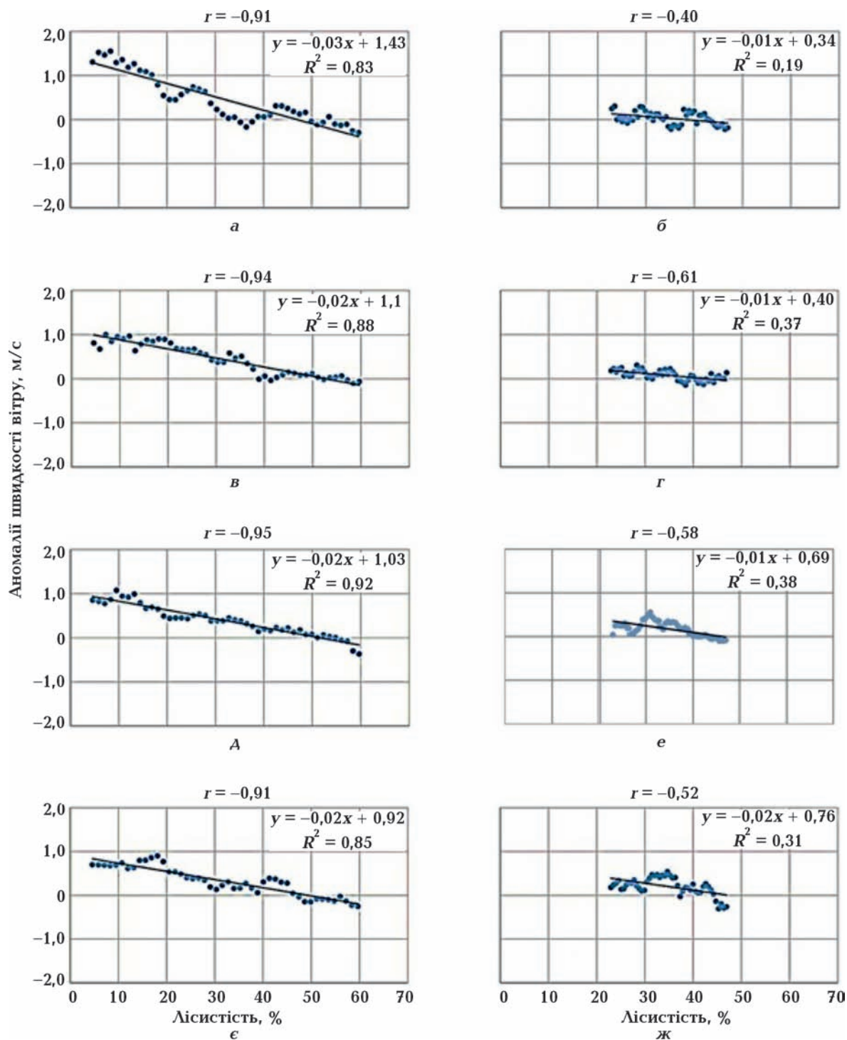
Рис. 5. Залежність зміни середньої місячної швидкості вітру (у м/с) від відсотка лісистості для північної широтної зони за ГКМ 5 (а) та ГКМ 6 (б) на прикладі січня, квітня (в) та (г), липня (А) та (е), жовтня (є) та (ж). Fig. 5. The dependence of the change in the mean monthly wind speed in m/s on the percentage of forest cover for the northern latitudinal zone on the examples of GCMs 5 (a), 6 (б) for January, for April (в) and (г), for July (А) and (е), for October (є) and (ж).
