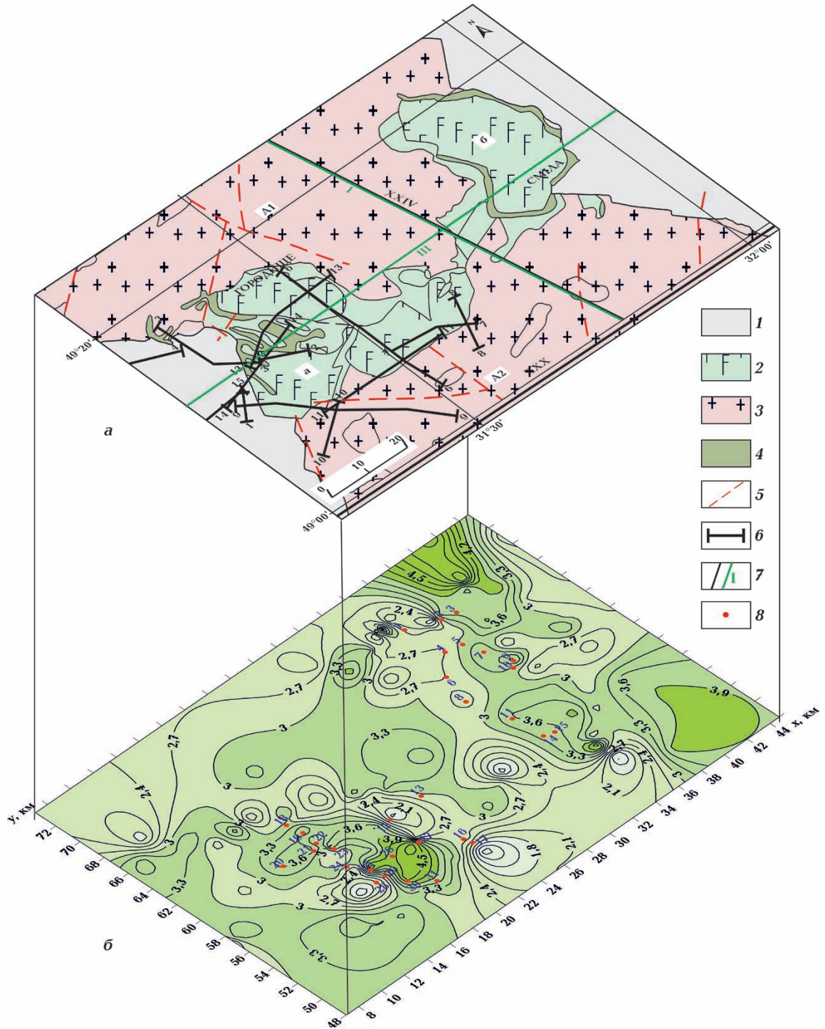
Рис. 5. Карта-схема: а — геологічної будови центральної частини Корсунь-Новомиргородського плутону; б — карта-схема ізогіпс глибин залягання нижньої кромки апроксимаційної моделі, одержаної в результаті розв'язання оберненої задачі; 1 — гнейси, 2 — граніти рапаківі, 3 — габро-анортозити, 4 — монзоніти, 5 — розломи, 6 — сейсмічні профілі СГТ, 7 — сейсмічні профілі ГСЗ і МОХЗ та їх номери, 8 — розташування об'єктів підібраної моделі.
