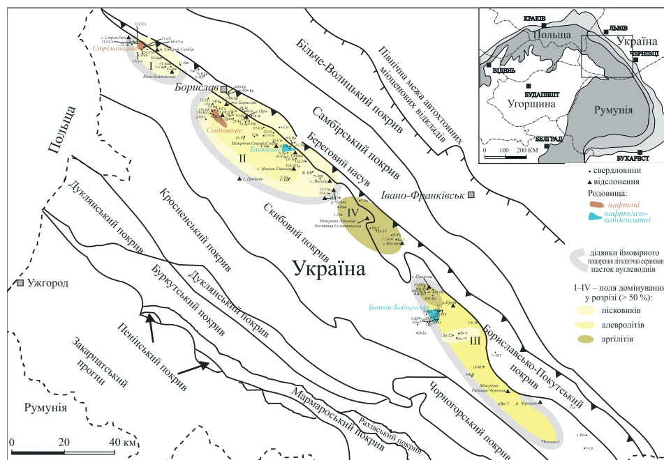
Рис. 8. Карта поширення полів перспективних порід-колекторів палеоценових відкладів у межах Берегової та Орівської скиб Українських Карпат. Геологічна будова за (Круглов та ін., 1985; Шакін та ін., 1977; Шлапінський, 2015)
