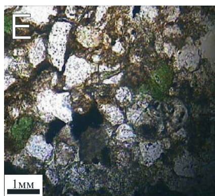
Рис. 3. Мікрофотографії порід палеоцену передових скиб Скибової зони Українських Карпат:
