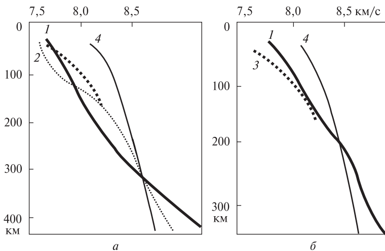
Рис. 10. Скоростные разрезы верхней мантии СОХ (А) и континентальной окраины атлантического типа (Б): 1 — экспериментальные скоростные разрезы, 2 — расчетный по АПГ скоростной разрез СОХ, 3 — значения V_p при температуре солидуса, 4 — скоростная модель докембрийской платформы
