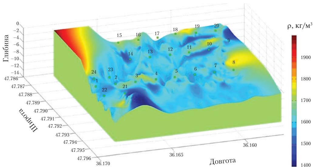
Рис. 2. 3D-візуалізація району обстеження, яка побудована за даними глибини з нанесеною інтерполяцією інтенсивності щільності з позначками точок пробовідбору
