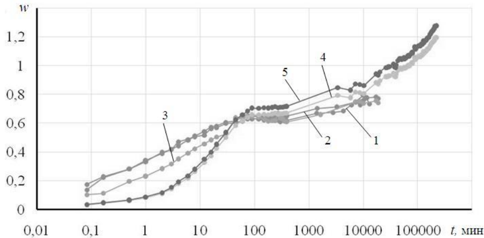
Рисунок 7 – Криві пропитки 6-го зразка пемзи в логарифмічному масштабі часу
