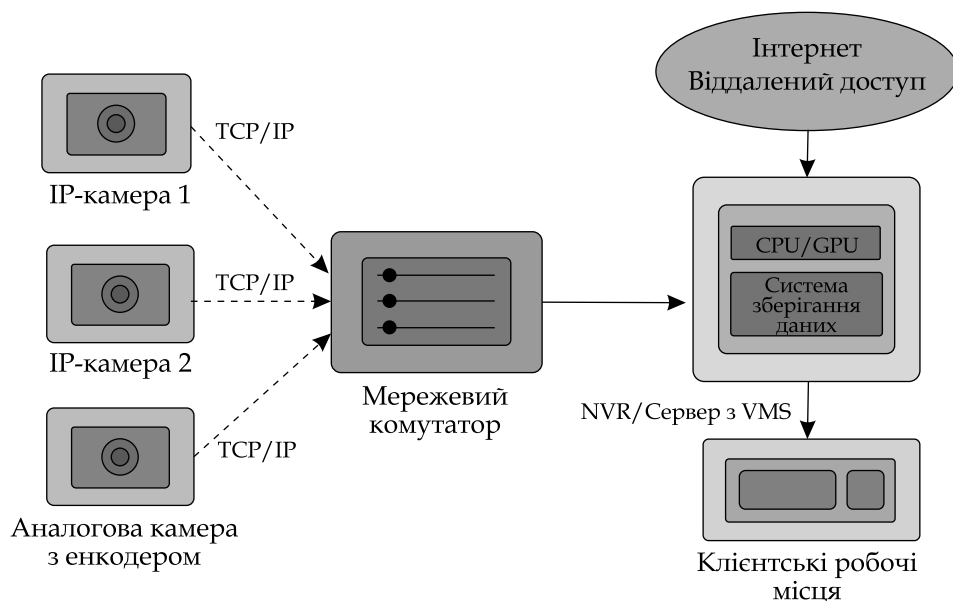
Рис. 2. Архітектура цифрової системи відеоспостереження [16]
