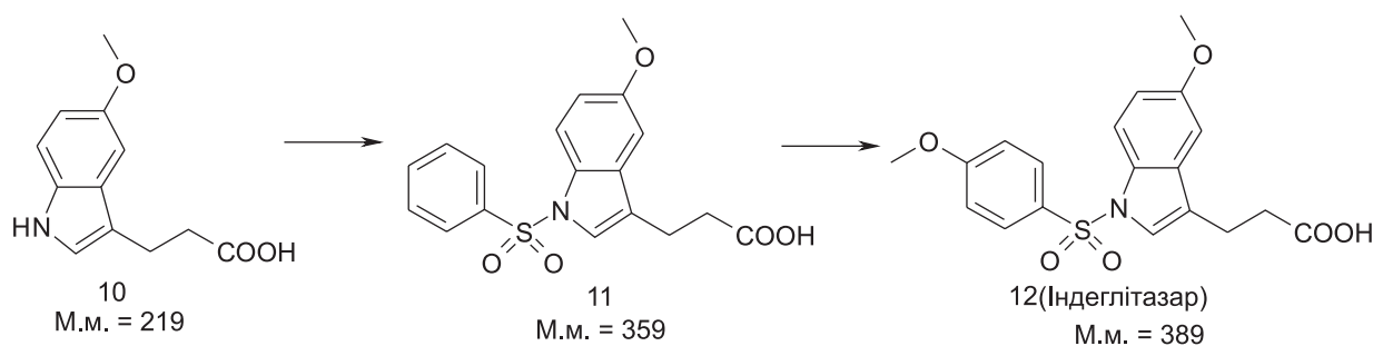
Рис. 16. Нарощування фрагменту при розробці Індеглітазару
