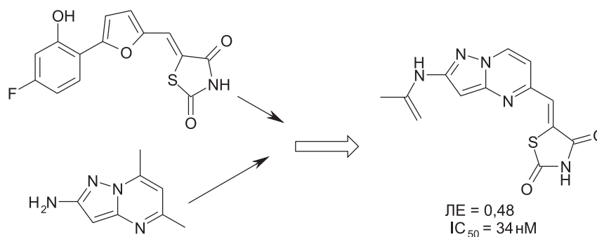
Рис. 9. Злиття імідазопіримідинових фрагментів з похідними тіазолідиндіону для одержання високоактивного інгібітора РІЗу кінази
