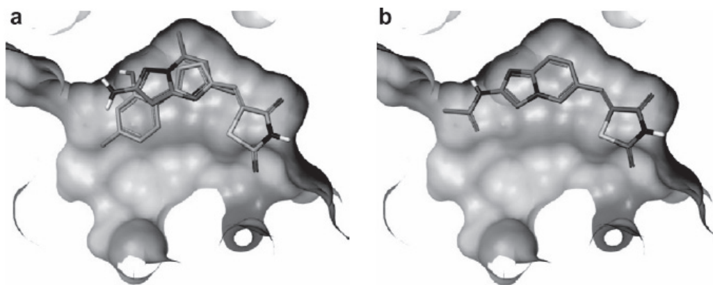
Рис. 10. а) накладання активного імідазопіримідинового фрагменту із тіазолідиндіоновим похідним; б) зв'язування гібридної сполуки з активним сайтом РІЗу кінази (адаптовано з [51])
