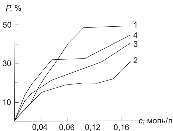
Рис. 3. Залежність ступеня розчинення фосфатних конкрементів від концентрації етилендіамінтетраацетату: 1 – перший шар; 2 – другий шар; 3 – третій шар; 4 – четвертий шар
