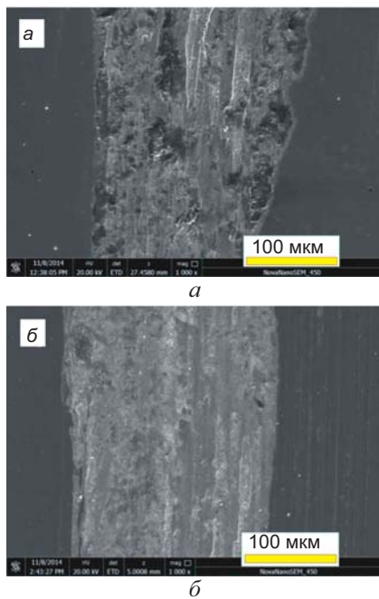
Рис. 24. РЕМ зображення структури доріжок тертя на поверхні покриття Ti-C-B, отриманого методом магнетронного розпорощення в парі з контртілом з Al 2 O 3 (а) і з контртіло з Ac100Cr6 (б)
