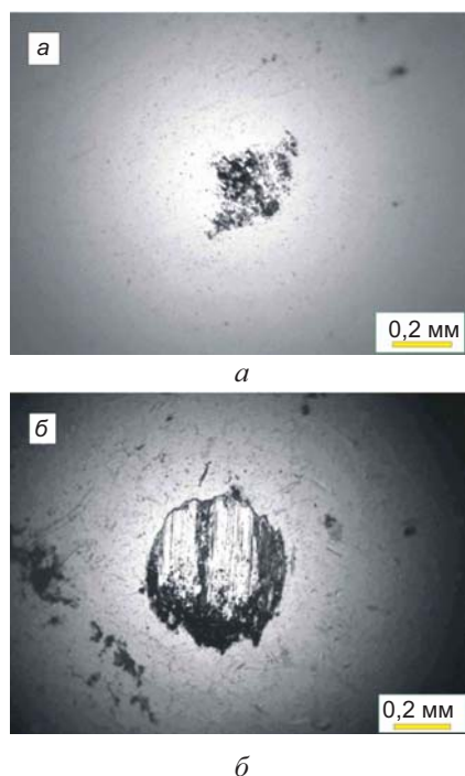
Рис. 19. Зображення плями зношування Al 2 O 3 (а) і сталі Ac100Cr6 (б) контргтіла після трибологічних досліджень покриттів Ti-B-C, отриманих методом магнетронного розпорошення
