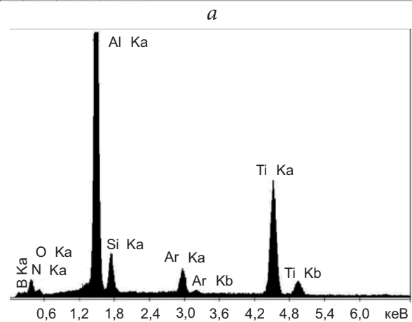
Рис. 3. Топографія поверхні покриття системи \text{AlN-TiB}_2\text{-TiSi}_2 : а) фрактограма зламу; РЕМ б) енергодисперсійний спектр
