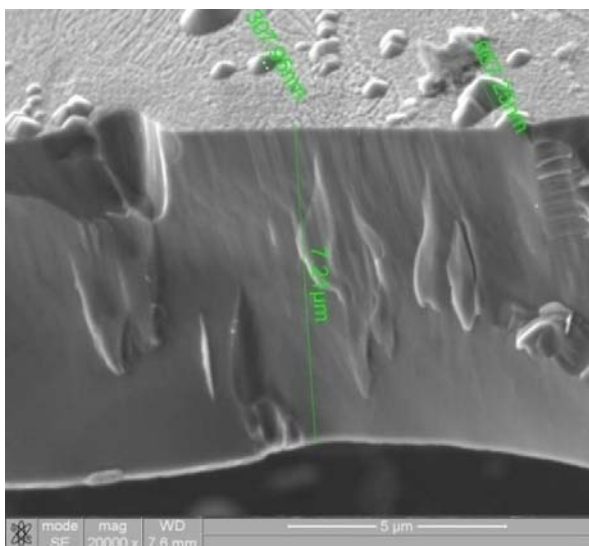
Рис. 2. Зображення фрактограми зламу покриття на основі системи AlN-(Ti-Cr)B 2 , отриманого при імпульсному магнетронному розпорощенні ( t — 95 хвилин)
