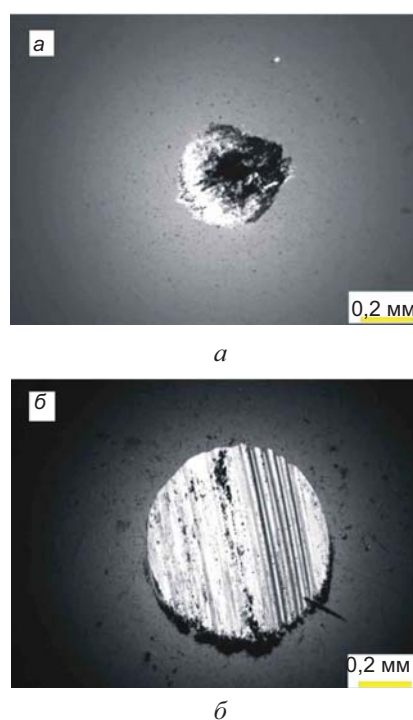
Рис. 20. Зображення плями зношування Al 2 O 3 (а) і сталі Ac100Cr6 (б) контргтіла після трибологічних досліджень покриттів Ti-B-C, отриманих методом вакуумно-дугового осадження
