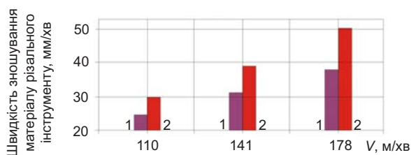
Рис. 25. Вплив швидкості різання на знос різців з покриттям AlN-TiB_2-TiSi_2 при точінні загартованої сталі ( s=0,1 мм/об; t=0,2 мм) ШХ15 (60 HRC): 1 — інструмент з покриттям; 2 — інструмент без покриття
