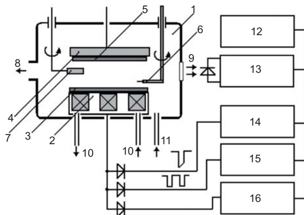
Рис. 1. Схема установки: 1 — вакуумна камера; 2 — планарний магнетрон; 3 — мішень, яка розпорошується; 4 — утримувач підкладки; 5 — підкладка; 6 — зонд Ленгмюра; 7 — кварцовий вимірювач товщини та швидкості осадження; 8 — система відкачування; 9 — оглядове вікно; 10 — водяне охолодження; 11 — напуск реакційного газу; 12 — система керування та запису даних; 13 — фотометр; 14 — блок живлення постійним струмом; 15 — блок живлення імпульсний; 16 — блок ВЧ живлення
