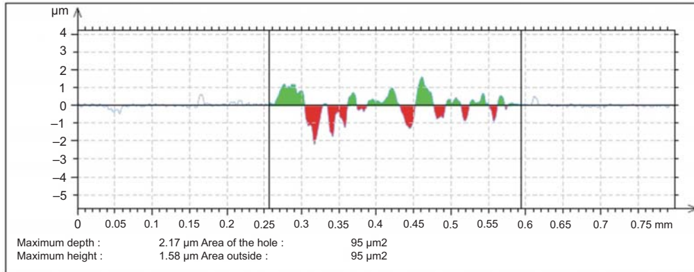
Рис. 21. Профілі поверхні, виміряні поперек доріжок тертя для покриття Ti-B-C, отриманого методом вакуумно-дугового осадження a ) для контртіла з \text{Al}_2\text{O}_3 ; б ) для контртіла з Ac100Cr6
