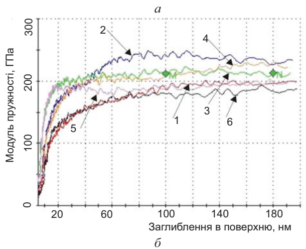
Рис. 5. Криві «навантаження-заглиблення» за глибиною при наноіндентуванні зразка покриття системи AlN-TiB_2-TiSi_2 : а) вимірювання твердості; б) вимірювання модуля пружності
