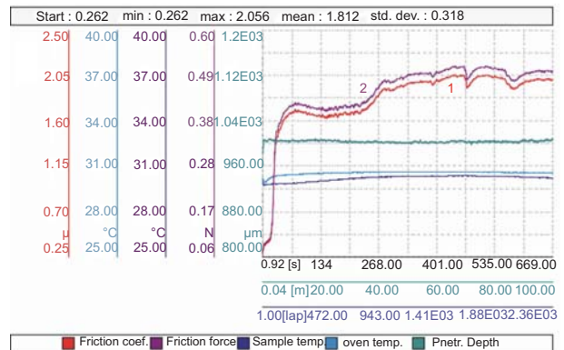
Рис. 18. Криві коефіцієнта тертя і сили тертя (чорвона (1) і фіолетова (2) лінії) для Ті-В-С покриттів, що наносяться методом імпульсного вакуумно-дугового (а) і ВЧ магнетронного розпорощення (б) з контртілом із Al_2O_3
