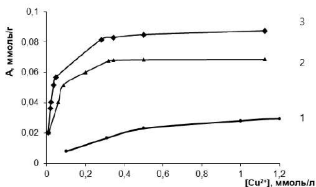
Рис. 8. Ізотерми сорбції йонів Cu(II) на поверхні немодифікованого вермикуліту (1), вермикуліту з in situ іммобілізованим (2) та з адсорбованим полі[8-оксихінолінметакрилатом] (3)
