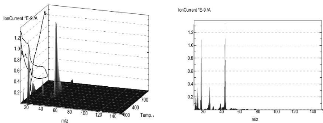
Рис. 5. Термограма вермикуліту з in situ іммобілізованим полі[8-оксихінолінметакрилатом], об'єднана з мас-спектром, у 3D форматі
