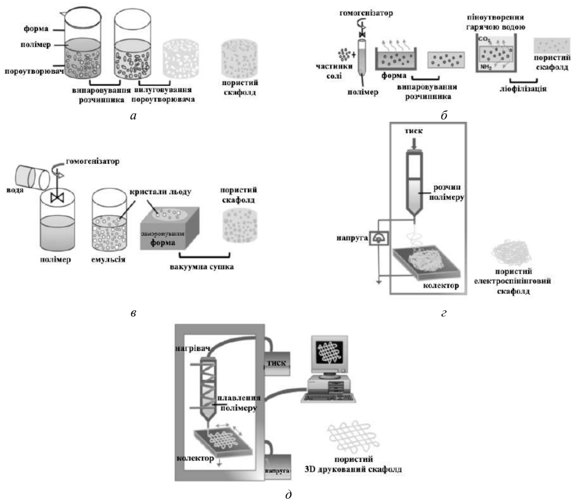
Рис. 2. Існуючі методи отримання БМ у вигляді пористих скафолдів: a – випаровування порогену, б – газове піноутворення, в – сублімація, г – електроспінінг розчину, д – електронапис та 3-D друк [7]
