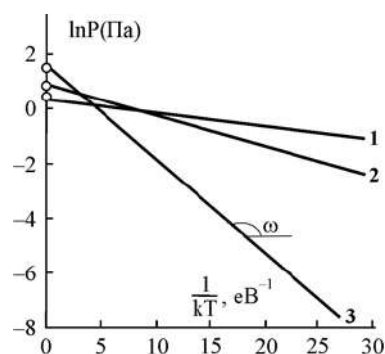
Рис. 4. Ізоплети розчинності водню в інтерметалідах MgYCo_4 , MgYCo_2Ni_2 , MgYNi_4 (прямі 1, 2, 3), побудовані за формулою (23) для \delta = \frac{1}{2} \delta_m і (1) c = 0.9 , U_{HH} = -0.6 eВ, (2) c = \frac{5}{6} , U_{HH} = -0.8 eВ, (3) c = \frac{2}{3} , U_{HH} = -1 eВ
