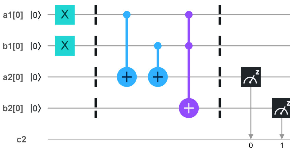
РИС. 3. Квантова схема для виконання складання двох кубіт з переносом розряду
